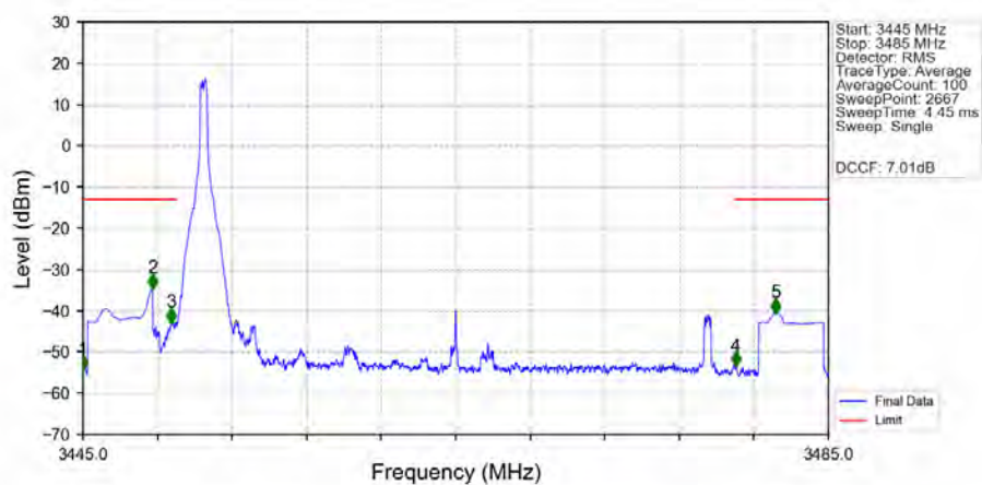
n78e_30kHz_SISO_NTNV_30MHz_DFT-s-OFDM_PI/2_BPSK_3465MHz_Inner_1RB_Left_Ant1
