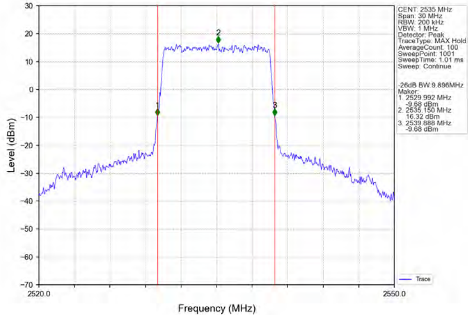
Band7_10MHz_QPSK_MCH_2535MHz_RB_50_0_NTNV
