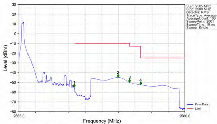
Band7_5MHz_QPSK_HCH_2567.5MHz_RB_1_24_NTNV
