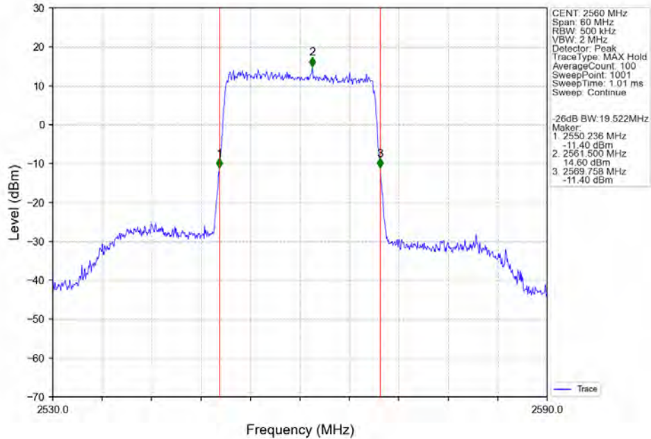
Band7_20MHz_256QAM_HCH_2560MHz_RB_100_0_NTNV
