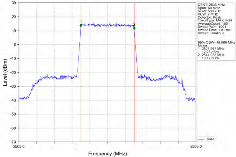
Band7_20MHz_QPSK_MCH_2535MHz_RB_100_0_NTNV
