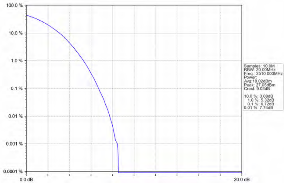
Band7_20MHz_256QAM_LCH_2510MHz_RB_100_0_NTNV
