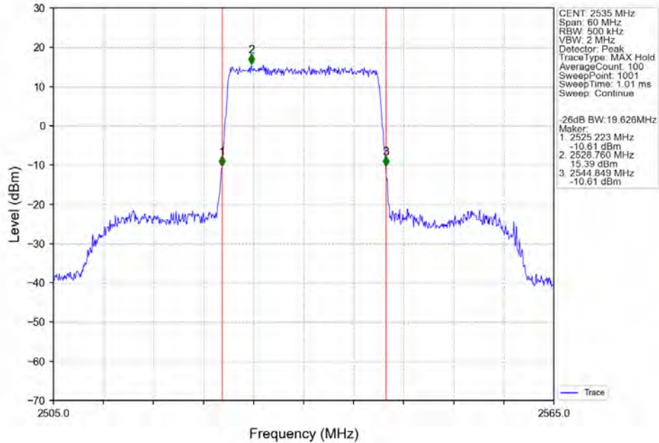
Band7_20MHz_QPSK_MCH_2535MHz_RB_100_0_NTNV
