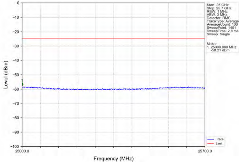
Band7_5MHz_QPSK_LCH_2502.5MHz_RB_1_0_NTNV
