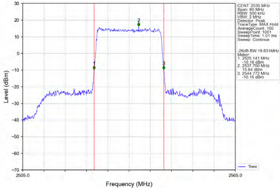
Band7_20MHz_64QAM_MCH_2535MHz_RB_100_0_NTNV
