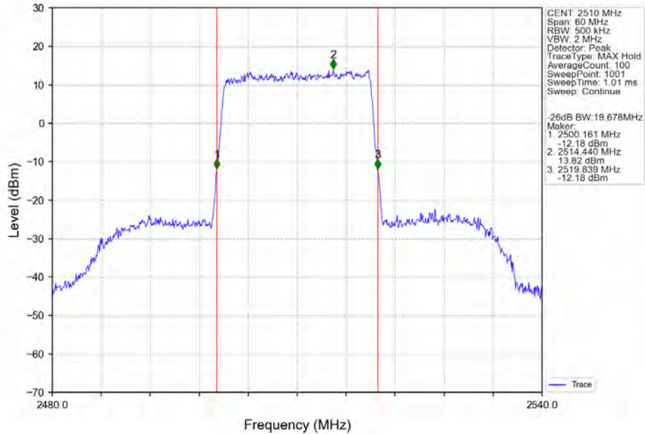
Band7_20MHz_256QAM_LCH_2510MHz_RB_100_0_NTNV
