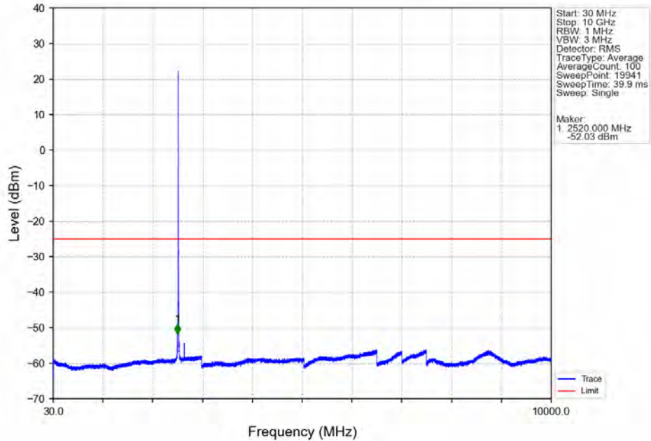
Band7_5MHz_QPSK_MCH_2535MHz_RB_1_0_NTNV
