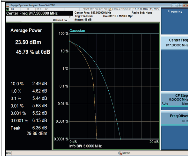
Band26(824-849)-3MHz-QPSK-27025-15RB#0-PASS
