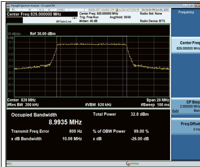
Band26(824-849)-10MHz-QPSK-26840-50RB#0-PASS
