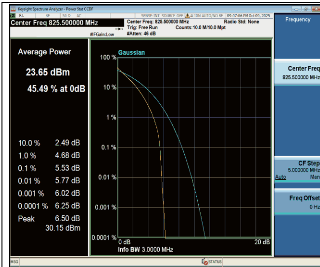
Band26(824-849)-3MHz-QPSK-26805-15RB#0-PASS
