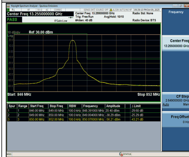
Band26(824-849)-10MHz-QPSK-26990-1RB#49-PASS
