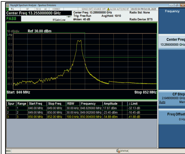
Band26(824-849)-3MHz-QPSK-27025-1RB#14-PASS
