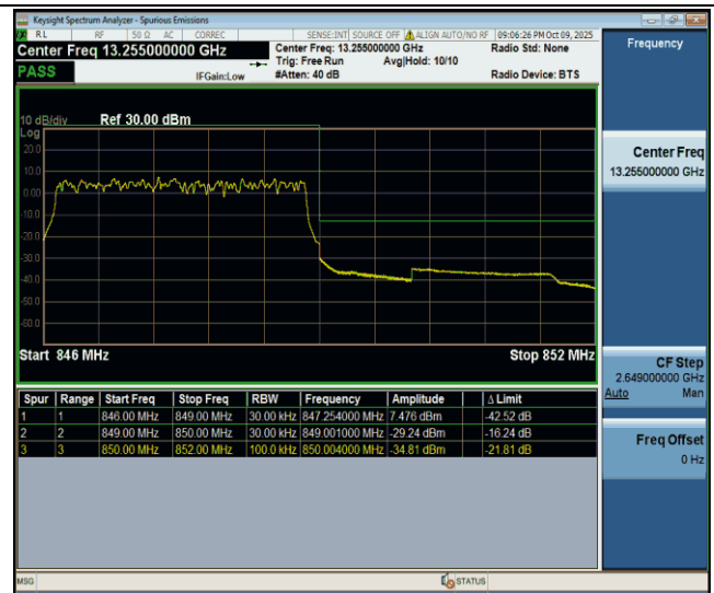
Band26(824-849)-3MHz-QPSK-27025-15RB#0-PASS
