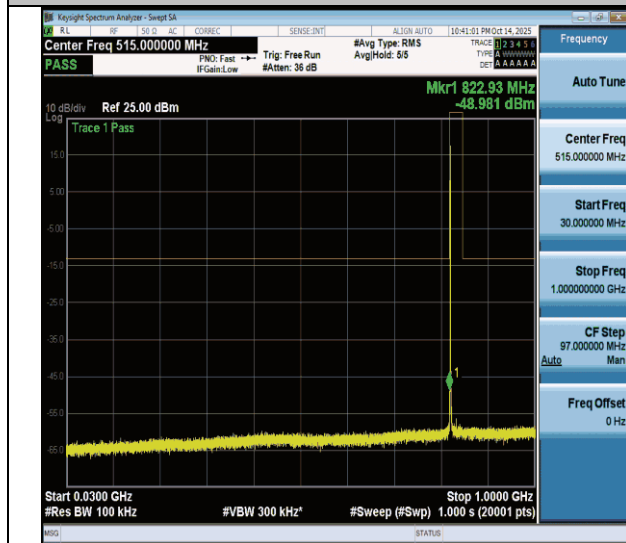
NTNV-n26(824-849)-PC3-15-20-L-CP-QPSK-Edge_1RB_Left-30- 1000-PASS
