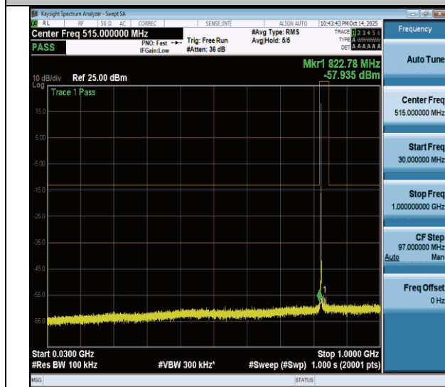
NTNV-n26(824-849)-PC3-15-20-M-CP-QPSK-Edge_1RB_Left-30- 1000-PASS
