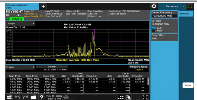
NTNV-Band14-10MHz-QPSK-23330-1RB#49--25.00--10.00-PASS
