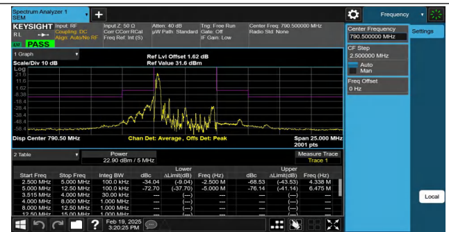
NTNV-Band14-5MHz-QPSK-23305-1RB#0--5.00--2.50-PASS
