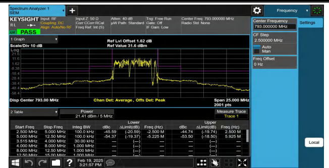
NTNV-Band14-5MHz-QPSK-23330-25RB#0--5.00--2.50-PASS
