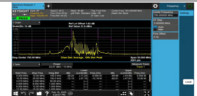
NTNV-Band14-10MHz-QPSK-23330-1RB#0--25.00--10.00-PASS
