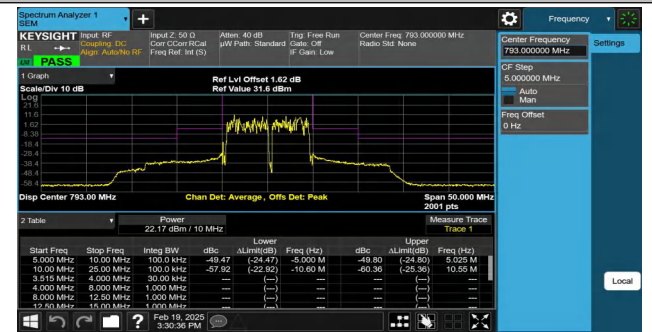
NTNV-Band14-10MHz-QPSK-23330-50RB#0--25.00--10.00-PASS
