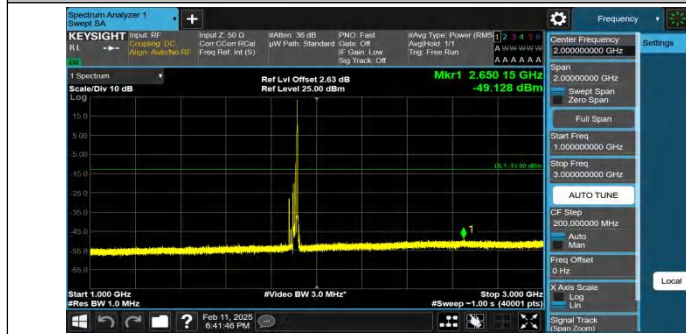
Band25-20MHz-QPSK-26590-1RB#99-1000~3000-PASS
