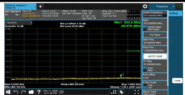
Band25-20MHz-QPSK-26590-1RB#99-30~1000-PASS
