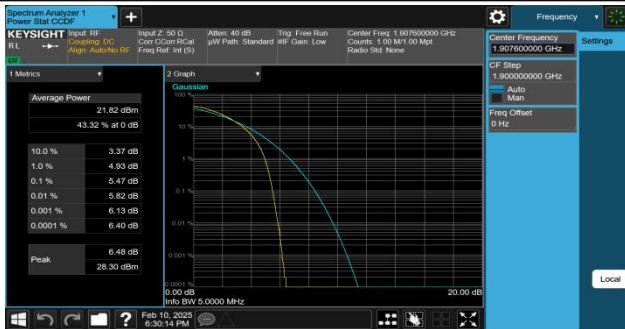
Band2-9538-3-PASS
