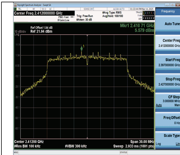
11n20SISO-Ant0-2412-0-Reference-PASS
