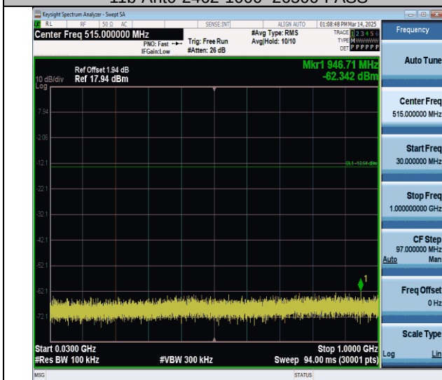
11g-Ant0-2412-30~1000-PASS
