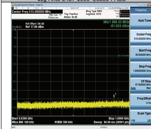
11g-Ant0-2462-30~1000-PASS
