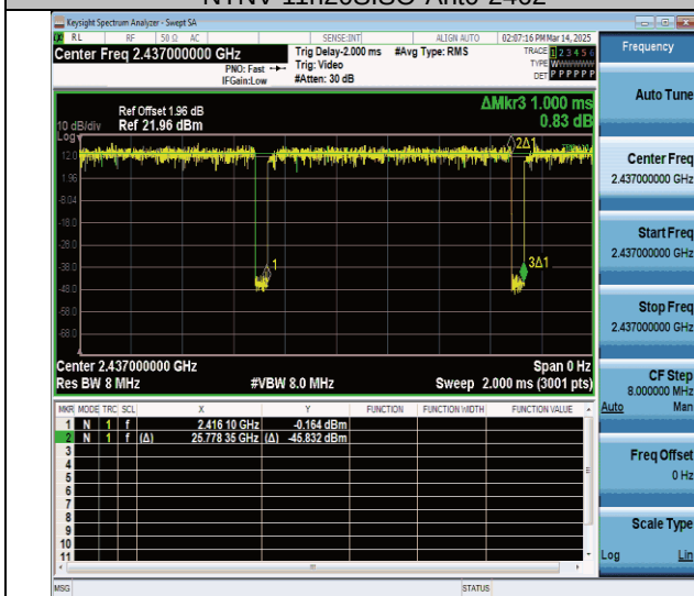
NTNV-11n40SISO-Ant0-2437
