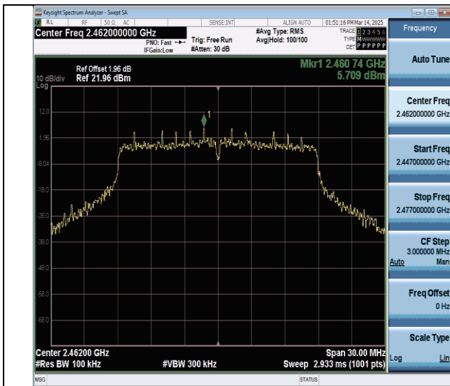
11n20SISO-Ant0-2462-0-Reference-PASS
