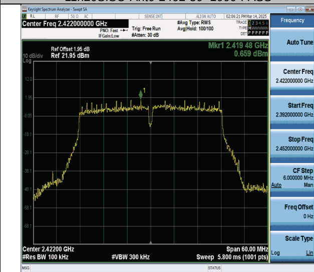
11n40SISO-Ant0-2422-0-Reference-PASS
