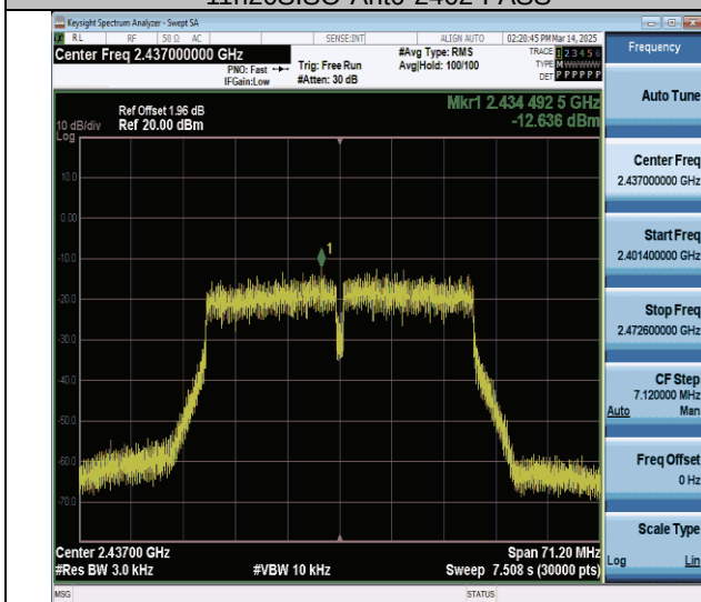
11n40SISO-Ant0-2437-PASS
