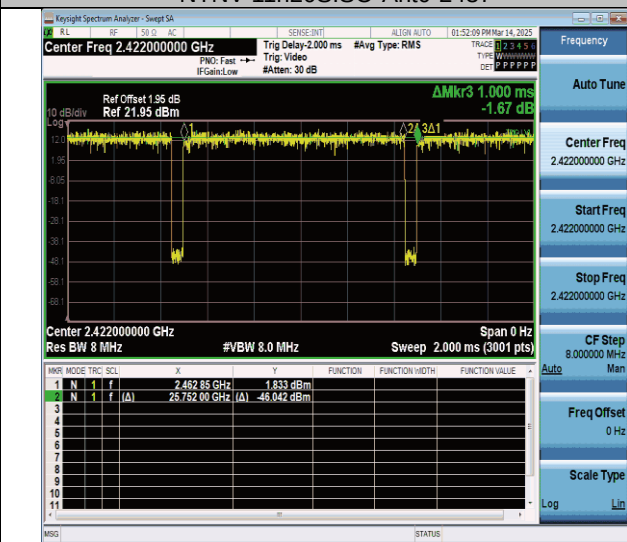
NTNV-11n40SISO-Ant0-2422
