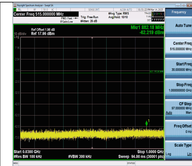
11n20SISO-Ant0-2462-30-1000-PASS
