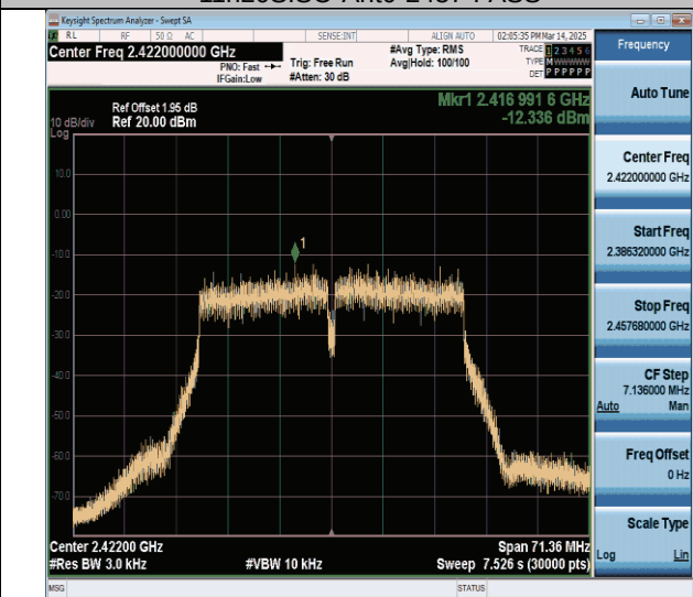
11n40SISO-Ant0-2422-PASS
