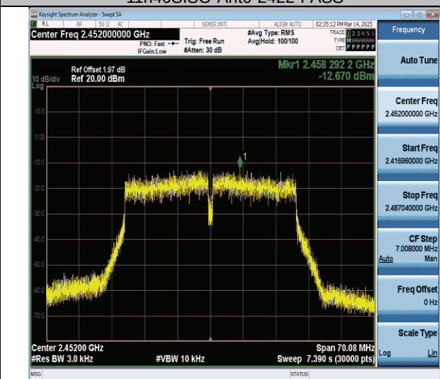
11n40SISO-Ant0-2452-PASS
