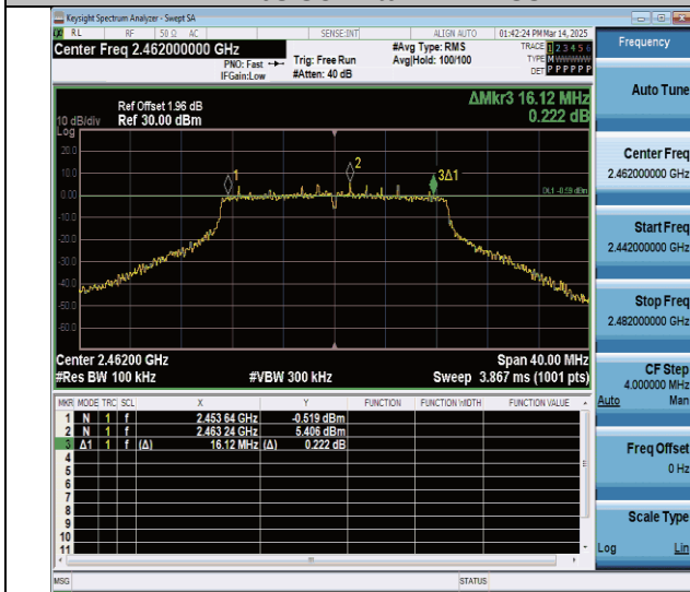
11n20SISO-Ant0-2462-PASS
