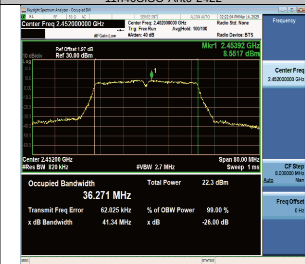
11n40SISO-Ant0-2452
