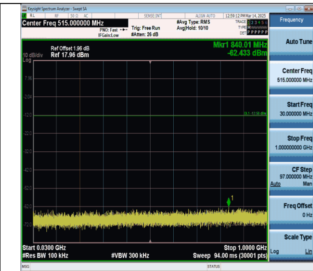
11b-Ant0-2462-30~1000-PASS
