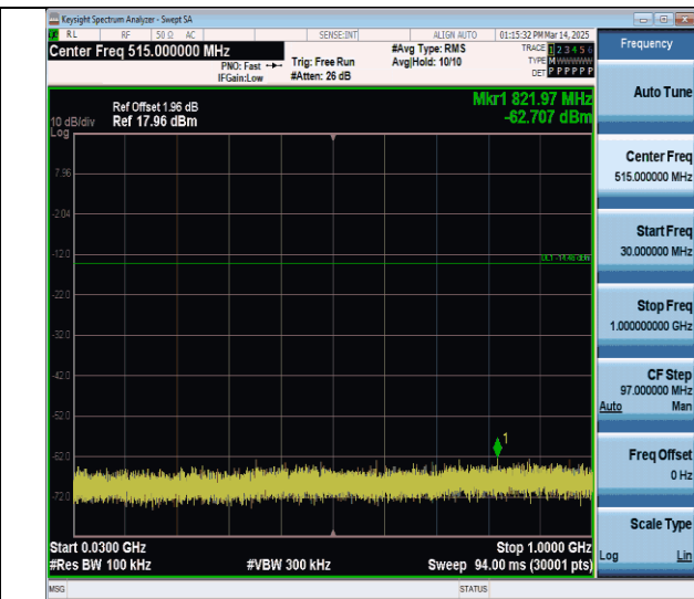
11g-Ant0-2437-30~1000-PASS
