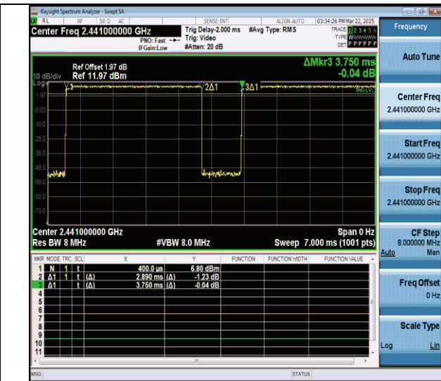
NTNV-3DH5-Ant0-2441
