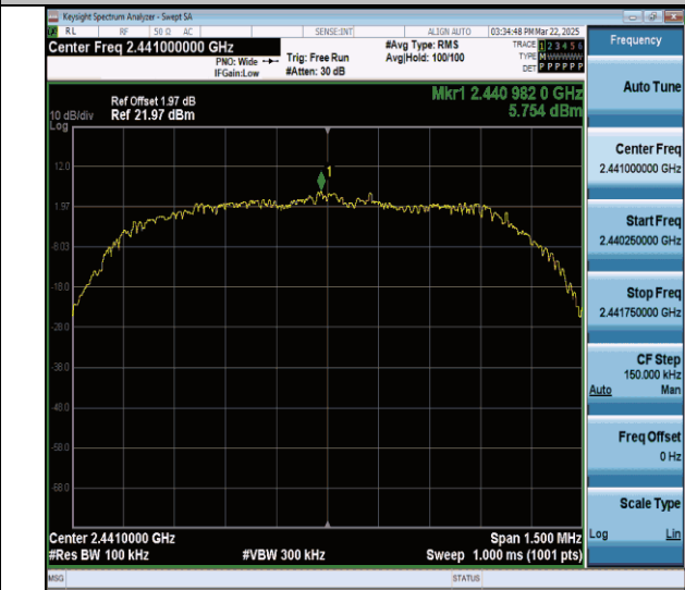
3DH5-Ant0-2441-0~Reference-PASS
