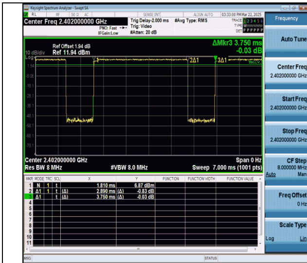
NTNV-3DH5-Ant0-2402
