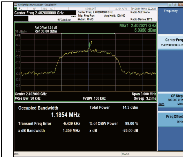
3DH5-Ant0-2402
