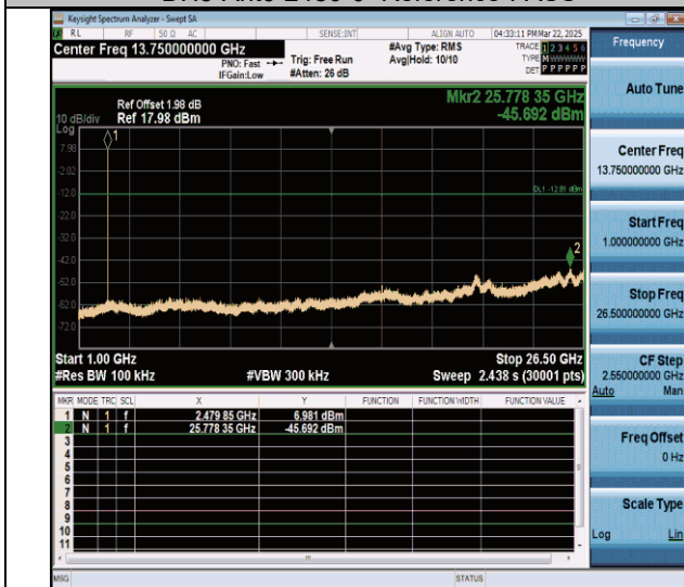
DH5-Ant0-2480-1000~26500-PASS
