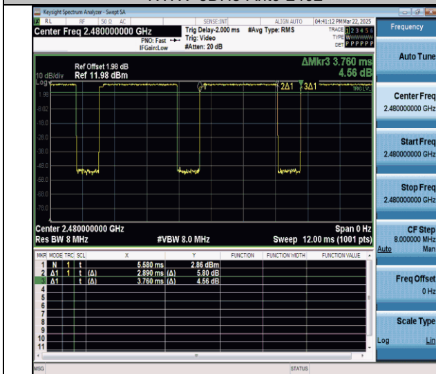
NTNV-3DH5-Ant0-2480
