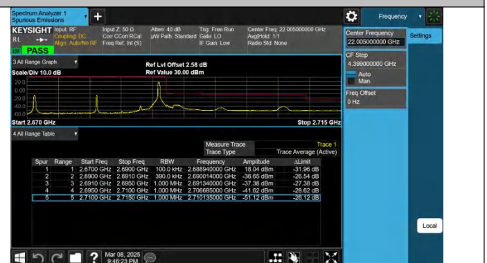
Band41-20MHz-QPSK-41490-1RB#99-PASS
