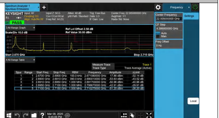
Band41-20MHz-QPSK-41490-1RB#0-PASS
