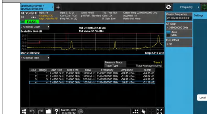
Band41-20MHz-QPSK-39750-1RB#99-PASS
