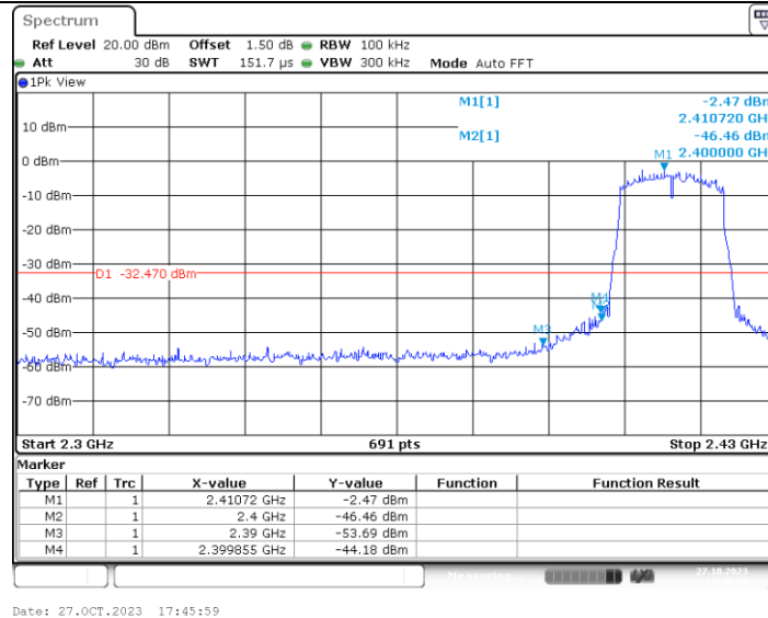
11N20MIMO_Ant4_Low_2412
