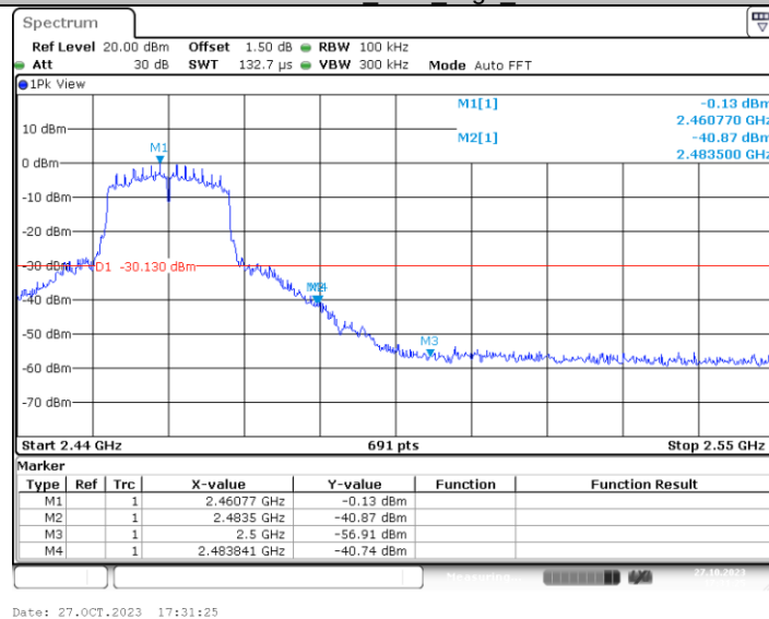
11N20MIMO_Ant4_High_2462
