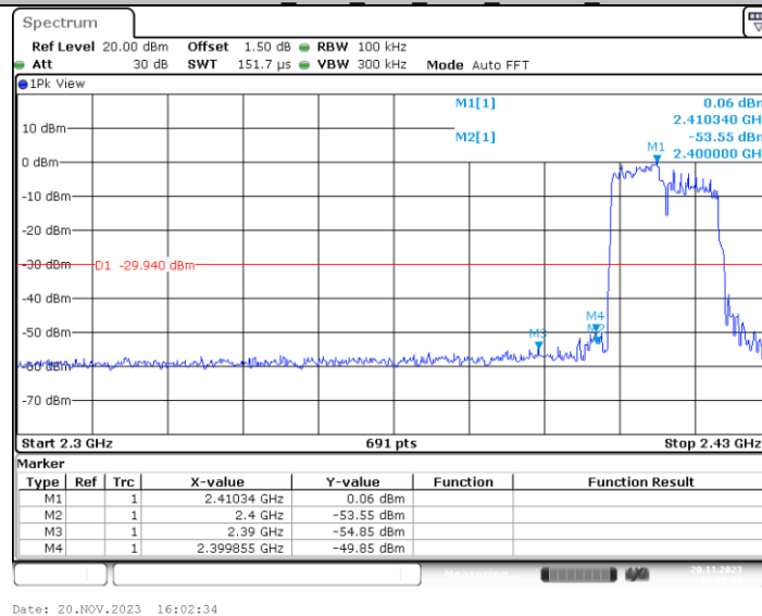
11AX20MIMO_Ant4_Low_2412_106Tone_RU53
