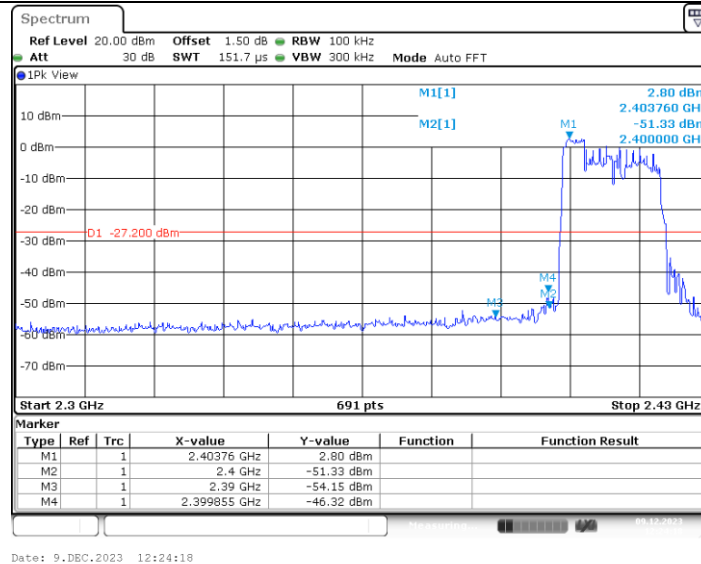
11AX20MIMO_Ant4_Low_2412_52Tone_RU37
