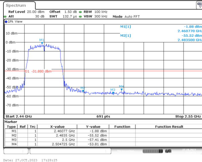
11N20MIMO_Ant3_High_2462
