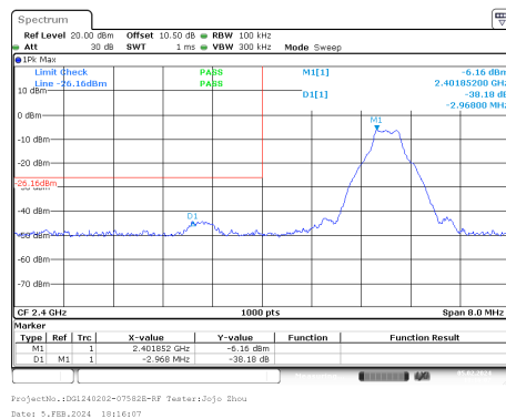
GFSK_Low_DH1
