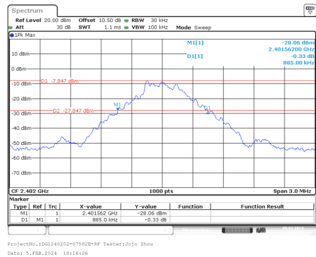
GFSK_Low_DH1
