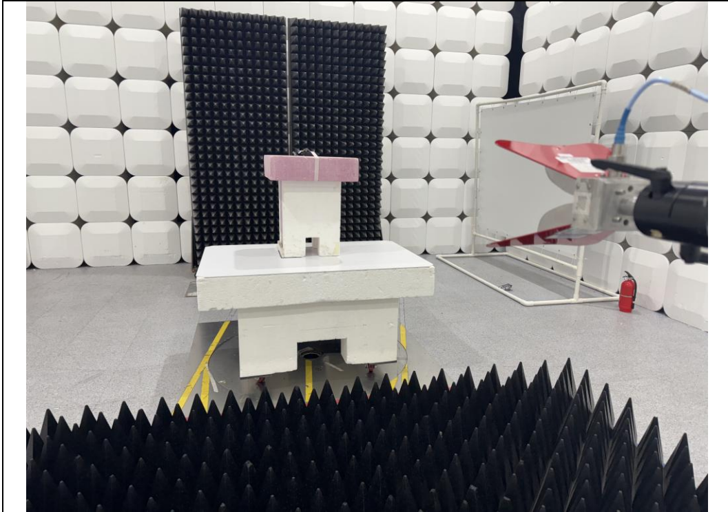
Test distance : 3 m, height of table : 1.5 m
