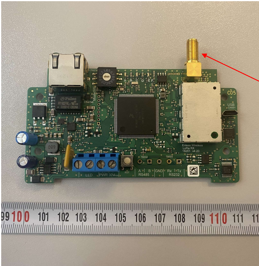
PCB bottom (600-501)
