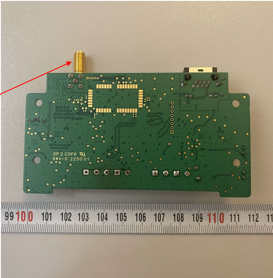
PCB bottom (600-501)
