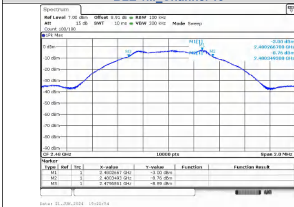
BLE 1M_Channel 39
