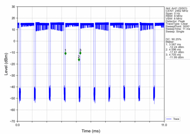
802.11b_HCH_2462MHz_Ant1 (SISO)_NTNV
