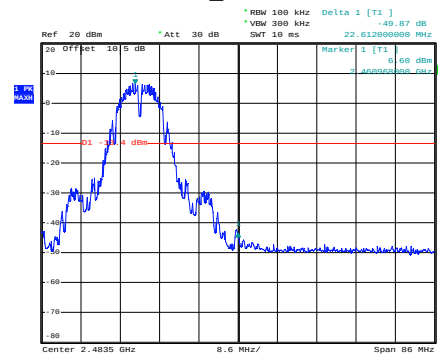
b_2462MHz
