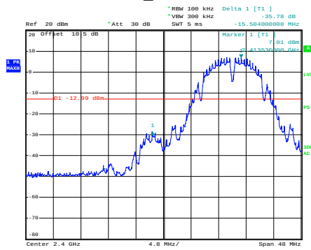
b_2412MHz
