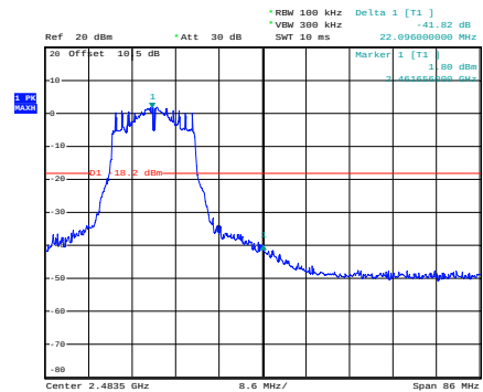
g_2462MHz
