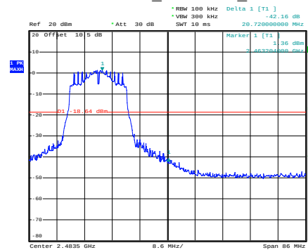
n20_2462MHz
