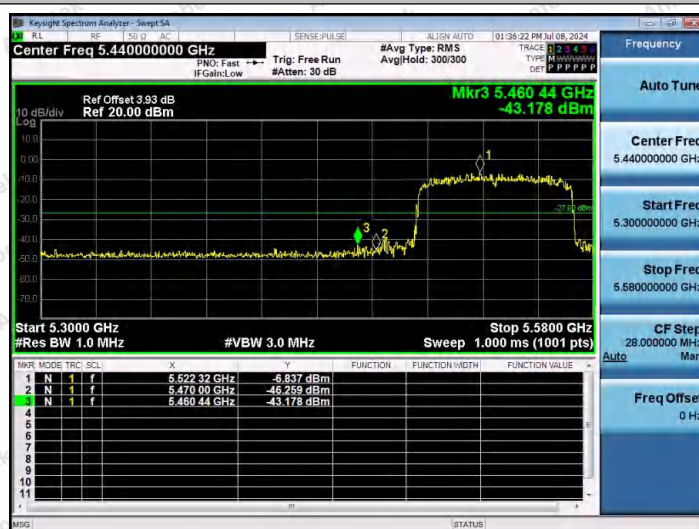
11AC80SISO-Ant1-5530-PASS
