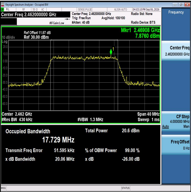
11N20MIMO-Ant1-2462
