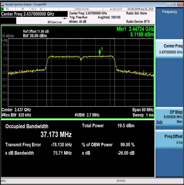
11N40MIMO-Ant2-2437
