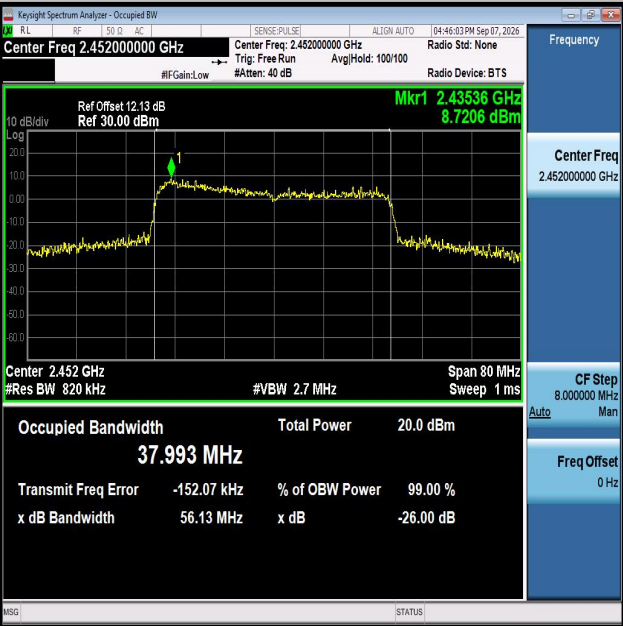
11AX40MIMO-Ant2-2452
