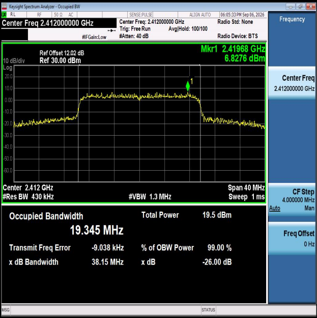
11AX20MIMO-Ant2-2412
