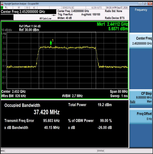
11AX40MIMO-Ant1-2452
