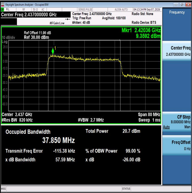
11AX40MIMO-Ant2-2437
