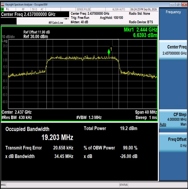
11AX20MIMO-Ant2-2437
