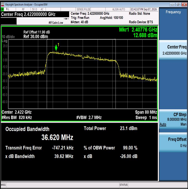
11AX40MIMO-Ant2-2422
