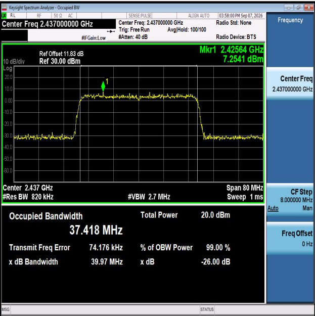
11AX40MIMO-Ant1-2437
