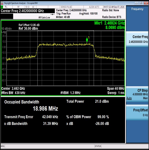
11AX20MIMO-Ant2-2462
