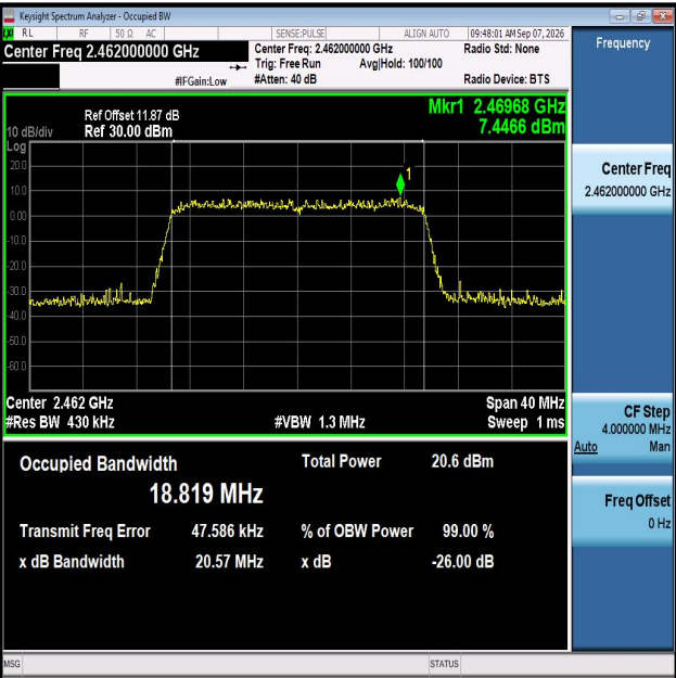
11AX20MIMO-Ant1-2462
