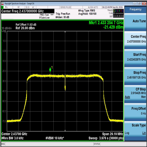
11AX20MIMO-Ant1-2437-PASS
