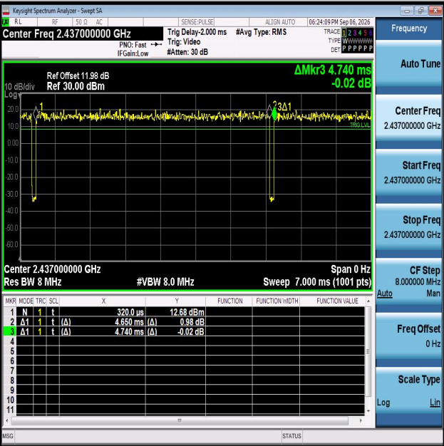
NTNV-11AX20MIMO-Ant2-2437
