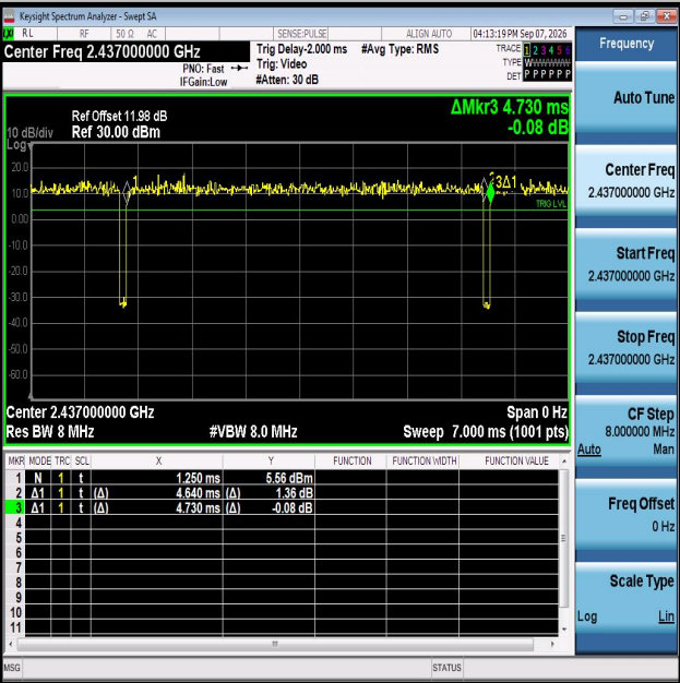
NTNV-11AX40MIMO-Ant2-2437
