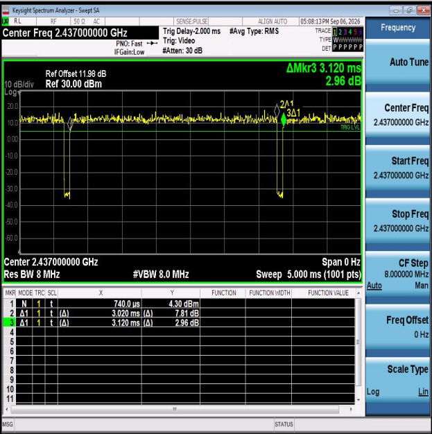
NTNV-11N40MIMO-Ant2-2437
