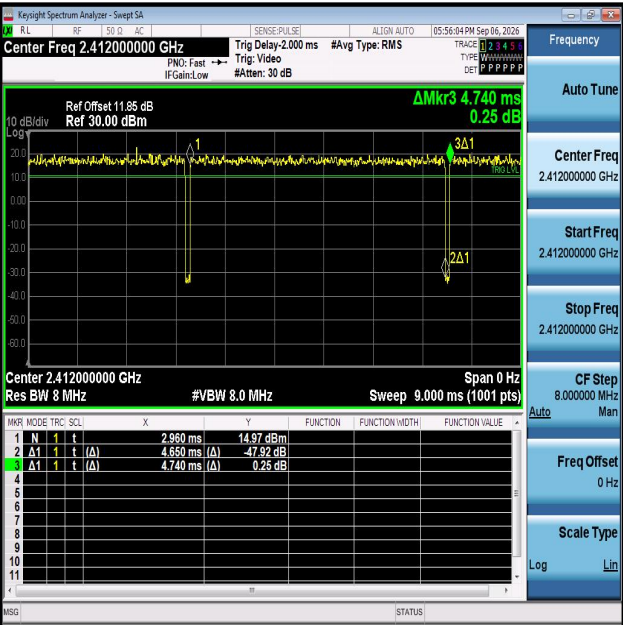
NTNV-11AX20MIMO-Ant1-2412
