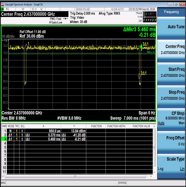
NTNV-11N20MIMO-Ant2-2437
