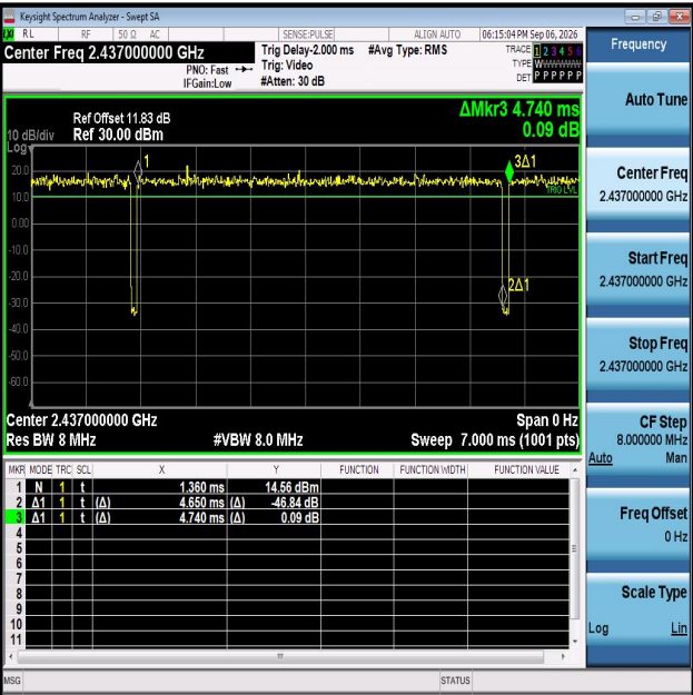
NTNV-11AX20MIMO-Ant1-2437
