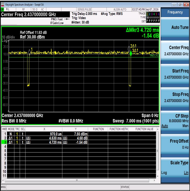
NTNV-11AX40MIMO-Ant1-2437
