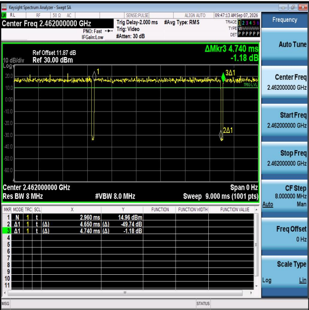
NTNV-11AX20MIMO-Ant1-2462
