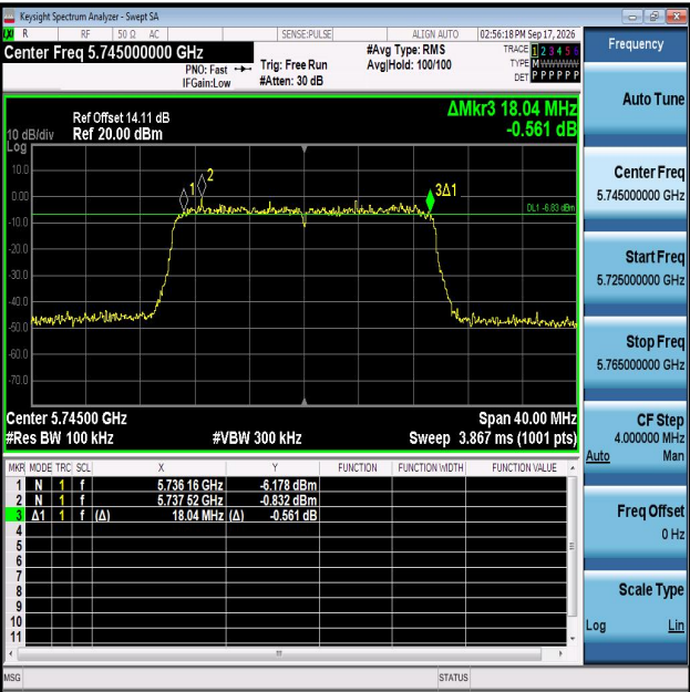
11AX20MIMO-Ant1-5745-PASS
