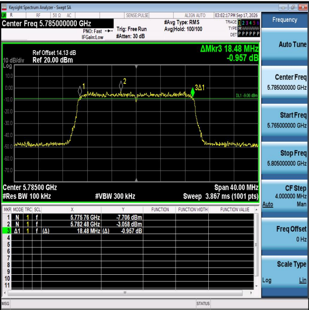
11AX20MIMO-Ant1-5785-PASS
