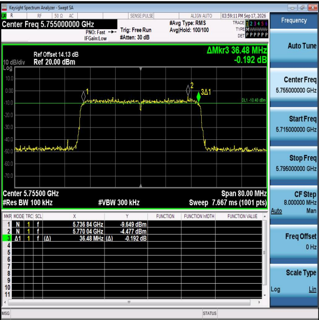
11AX40MIMO-Ant1-5755-PASS
