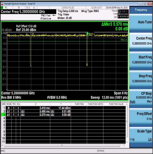
NTNV-11A-Ant1-5280
