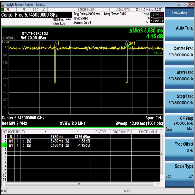
NTNV-11A-Ant1-5745
