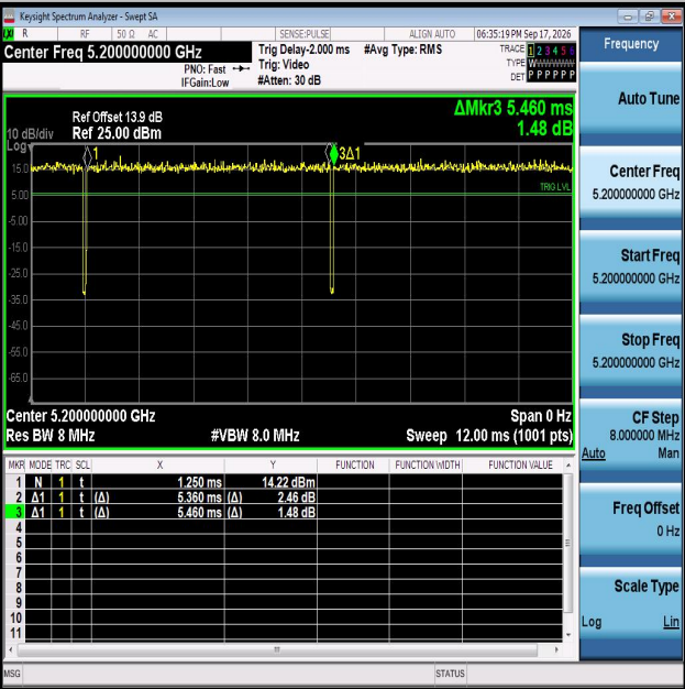
NTNV-11N20MIMO-Ant2-5200
