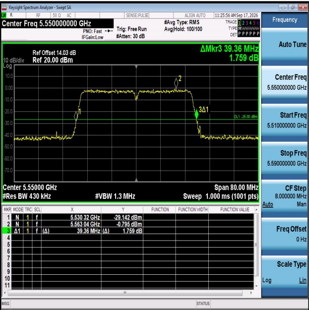
11AC40MIMO-Ant1-5550
