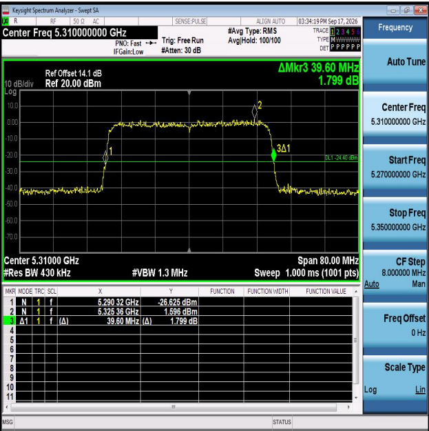
11AX40MIMO-Ant1-5310
