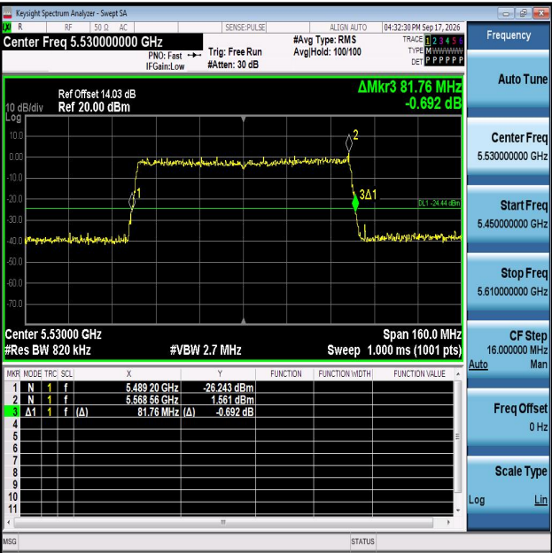
11AX80MIMO-Ant1-5530
