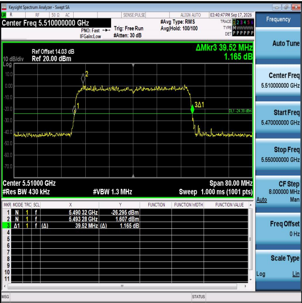
11AX40MIMO-Ant1-5510
