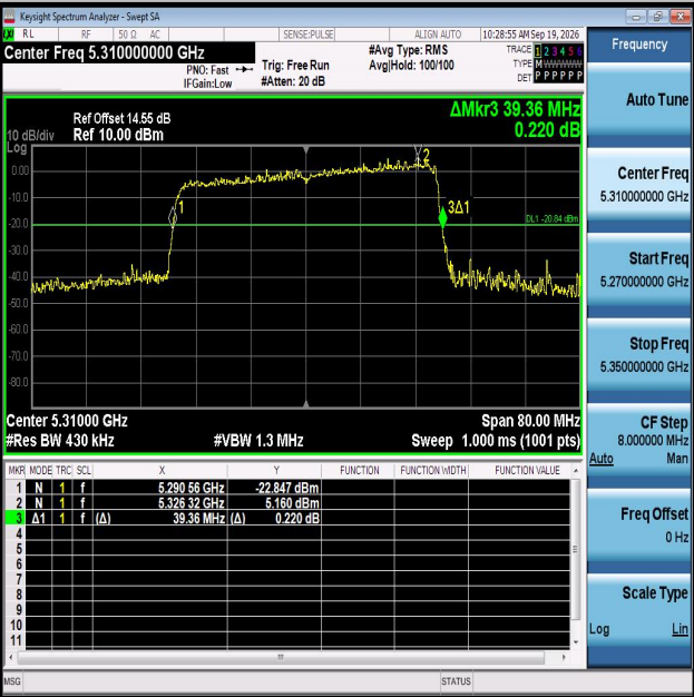
11AX40MIMO-Ant2-5310
