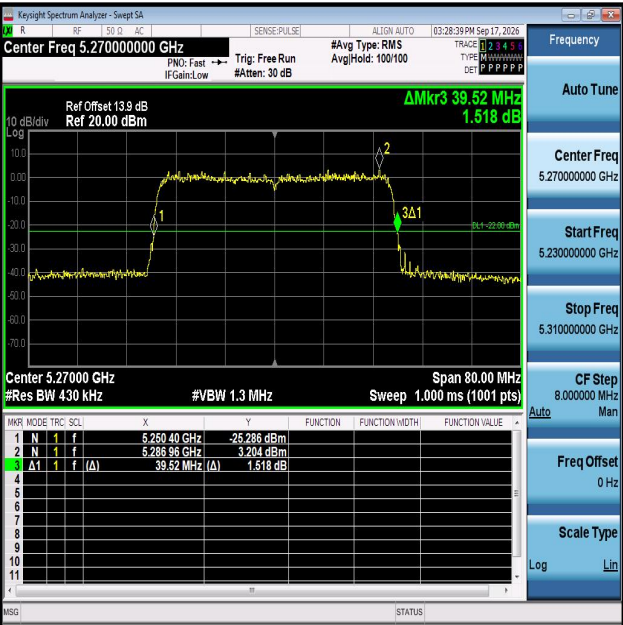
11AX40MIMO-Ant1-5270
