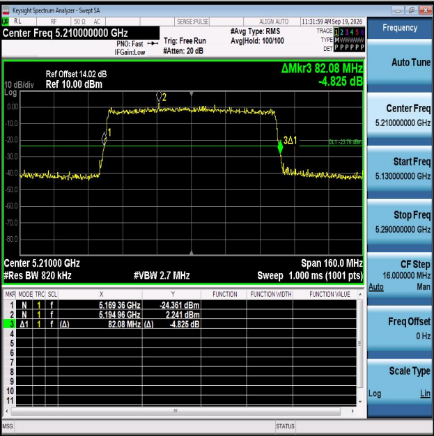
11AX80MIMO-Ant2-5210
