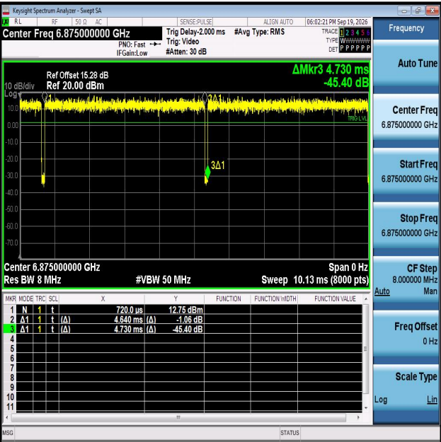
NTNV-11AX20MIMO-Ant1-6875
