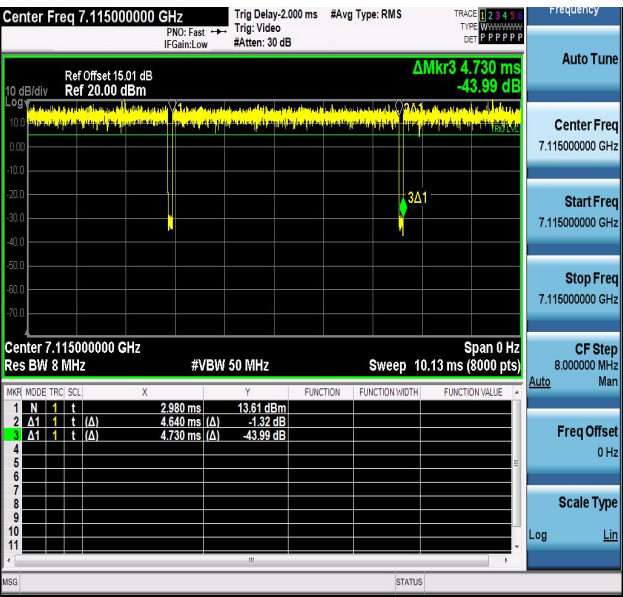
NTNV-11AX20MIMO-Ant2-7115
