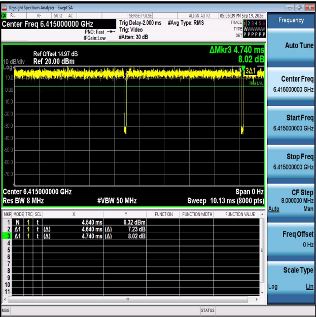
NTNV-11AX20MIMO-Ant1-6415
