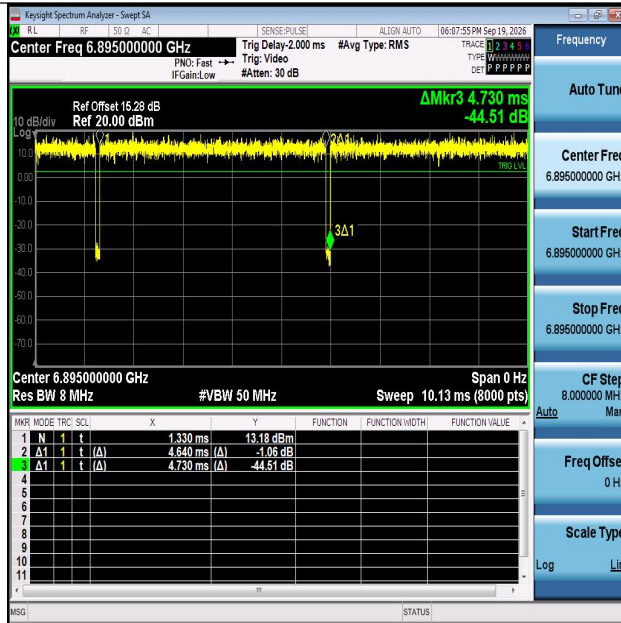
NTNV-11AX20MIMO-Ant1-6895
