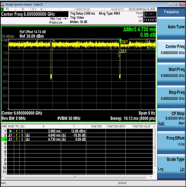
NTNV-11AX20MIMO-Ant1-6695
