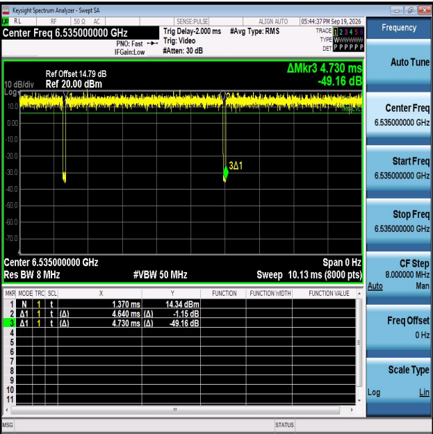
NTNV-11AX20MIMO-Ant1-6535
