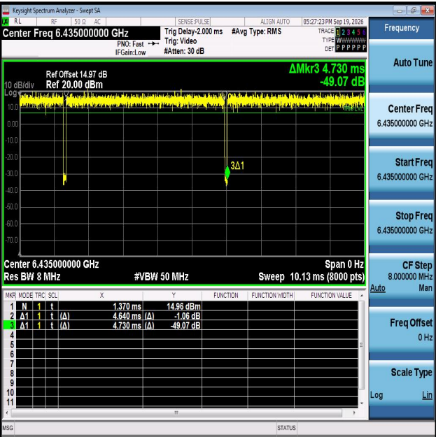
NTNV-11AX20MIMO-Ant1-6435
