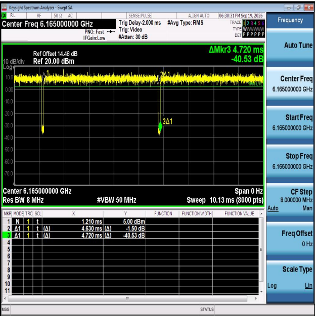
NTNV-11AX40MIMO-Ant1-6165
