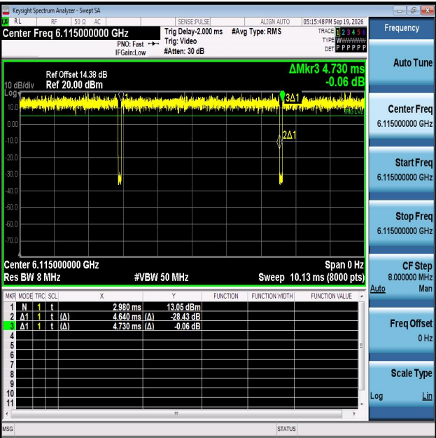
NTNV-11AX20MIMO-Ant1-6115
