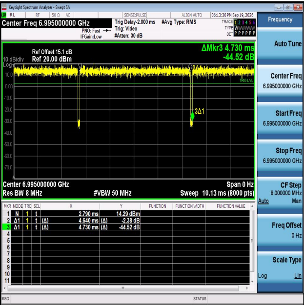
NTNV-11AX20MIMO-Ant1-6995
