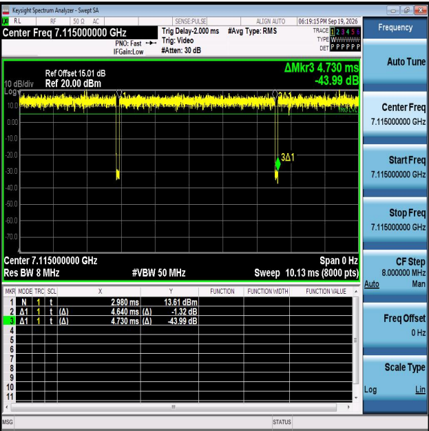
NTNV-11AX20MIMO-Ant1-7115
