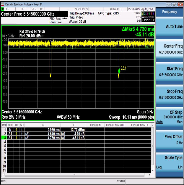
NTNV-11AX20MIMO-Ant1-6515
