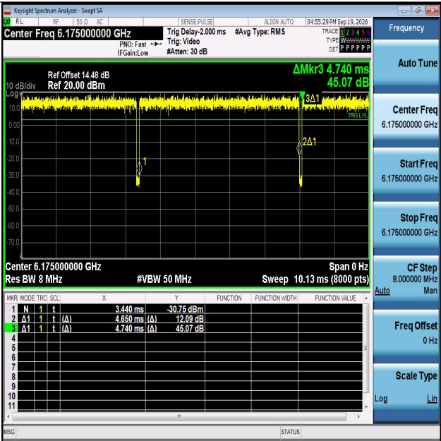
NTNV-11AX20MIMO-Ant1-6175
