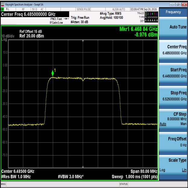
11AX40MIMO-Ant1-6485-PASS
