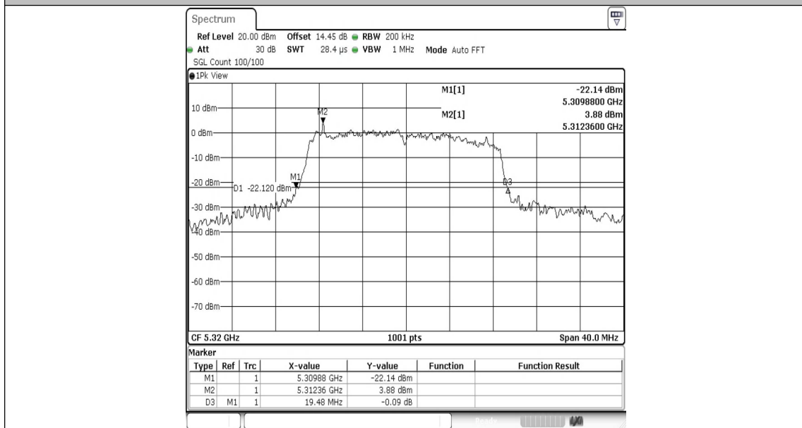
11N20MIMO-Ant1-5320
