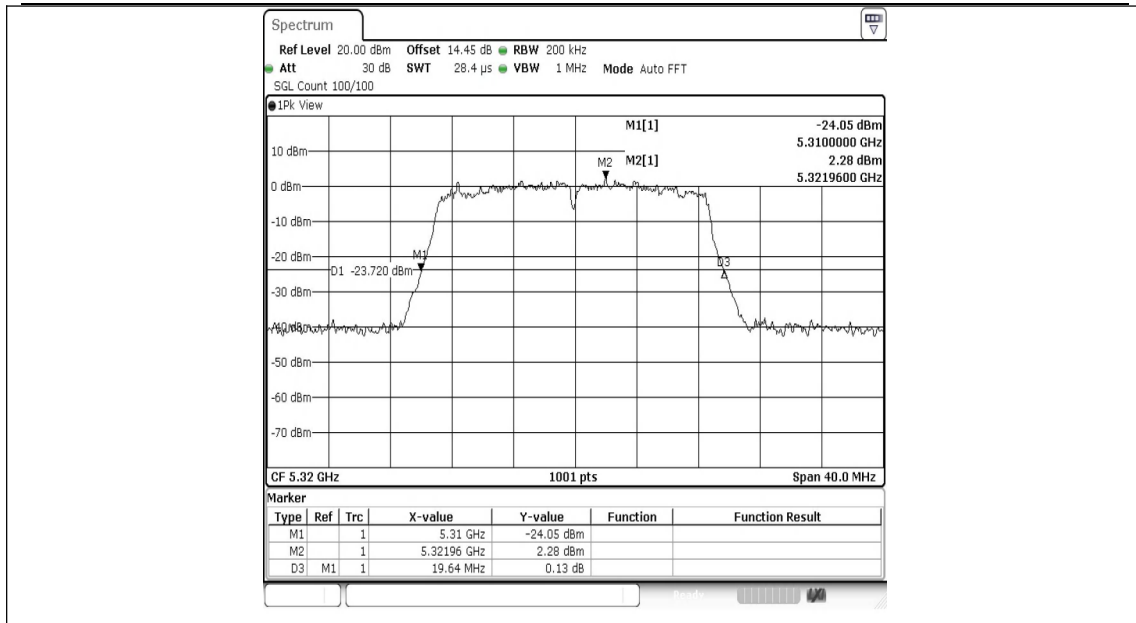
11N20MIMO-Ant1-5320
