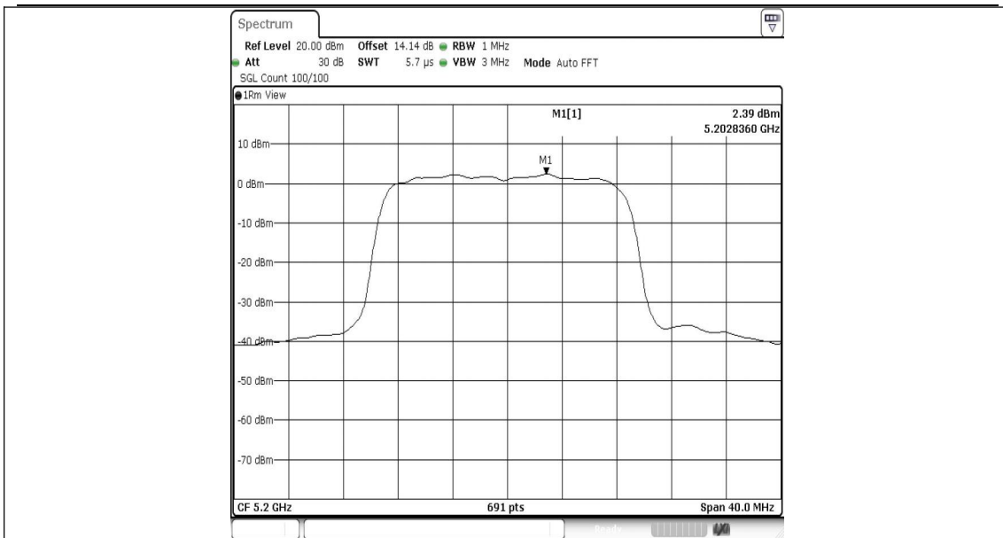
11N20MIMO-Ant1-5200-PASS
