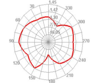
2450.000MHz E2
