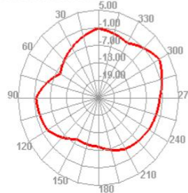
2500.000MHz H
