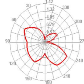
2400.000MHz E1
