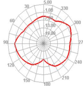
2450.000MHz H
