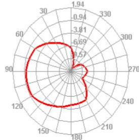
2500.000MHz E1
