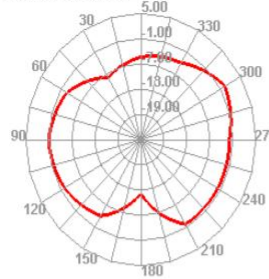
2400.000MHz H
