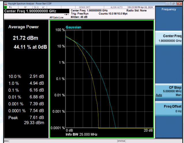
Band2-20MHz-16QAM-19100-27RB#0-PASS
