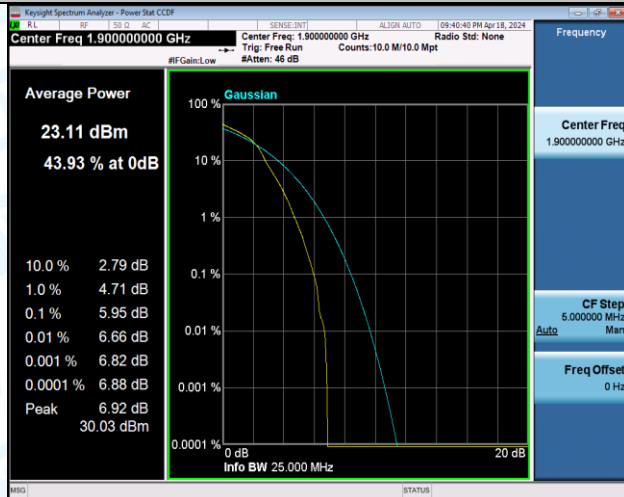
Band2-20MHz-16QAM-19100-1RB#0-PASS
