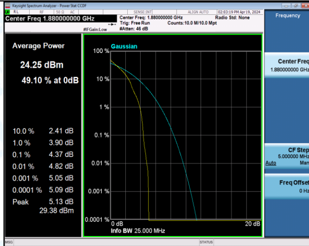
Band2-20MHz-QPSK-19100-1RB#0-PASS
