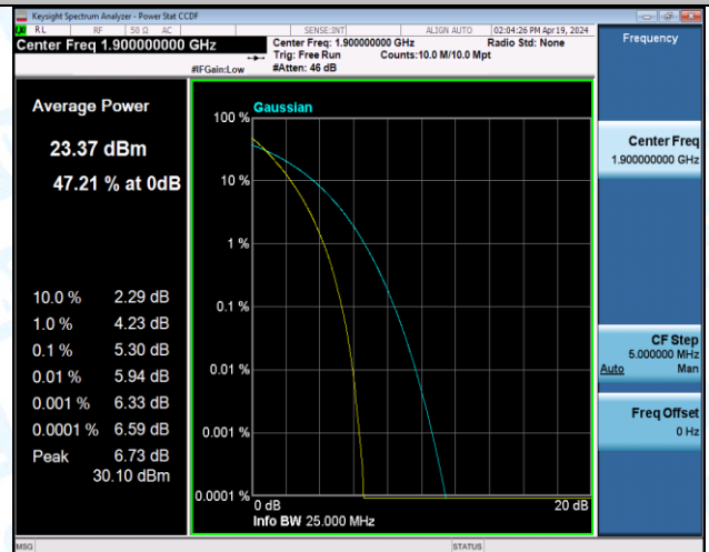
Band2-20MHz-16QAM-18700-27RB#0-PASS
