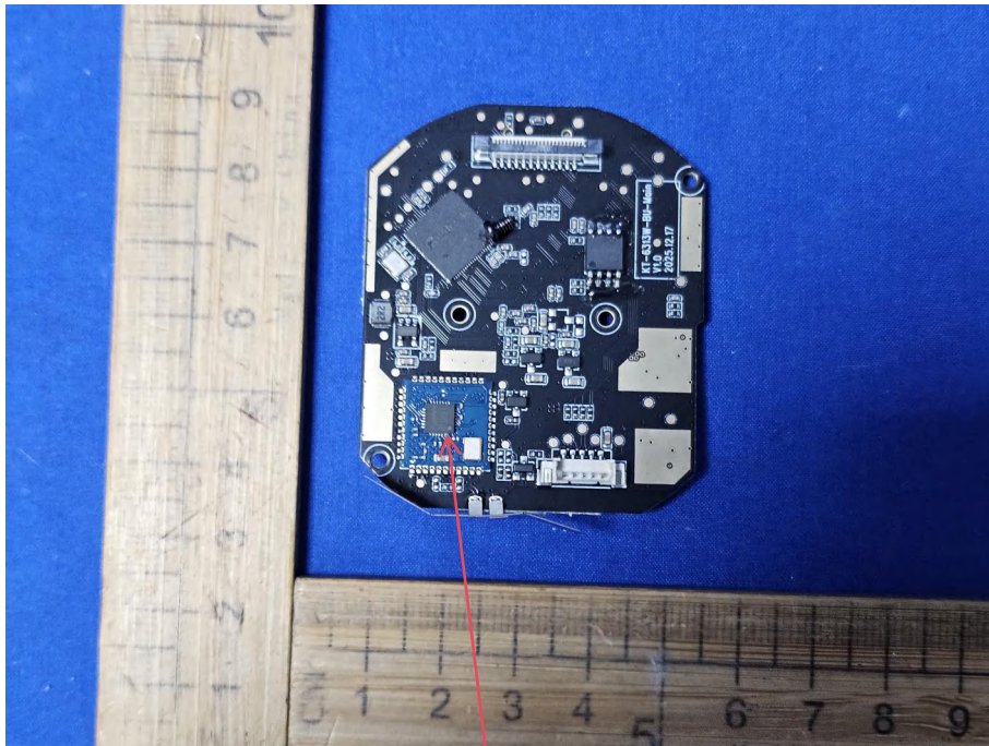
AB6032Is module
