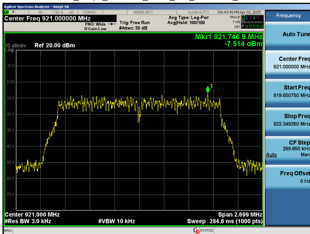
Test_Graph_802.11ah_ANT1_921_BW 2MHz_ PSD
