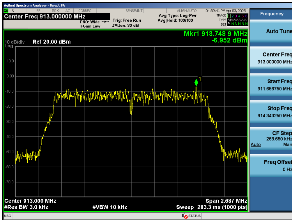
Test_Graph_802.11ah_ANT1_913_BW 2MHz_ PSD
