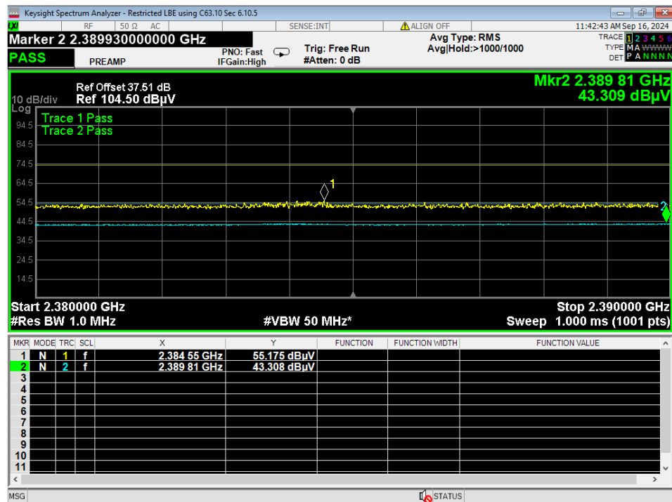
12 LBE Restricted, BLE 1MB
