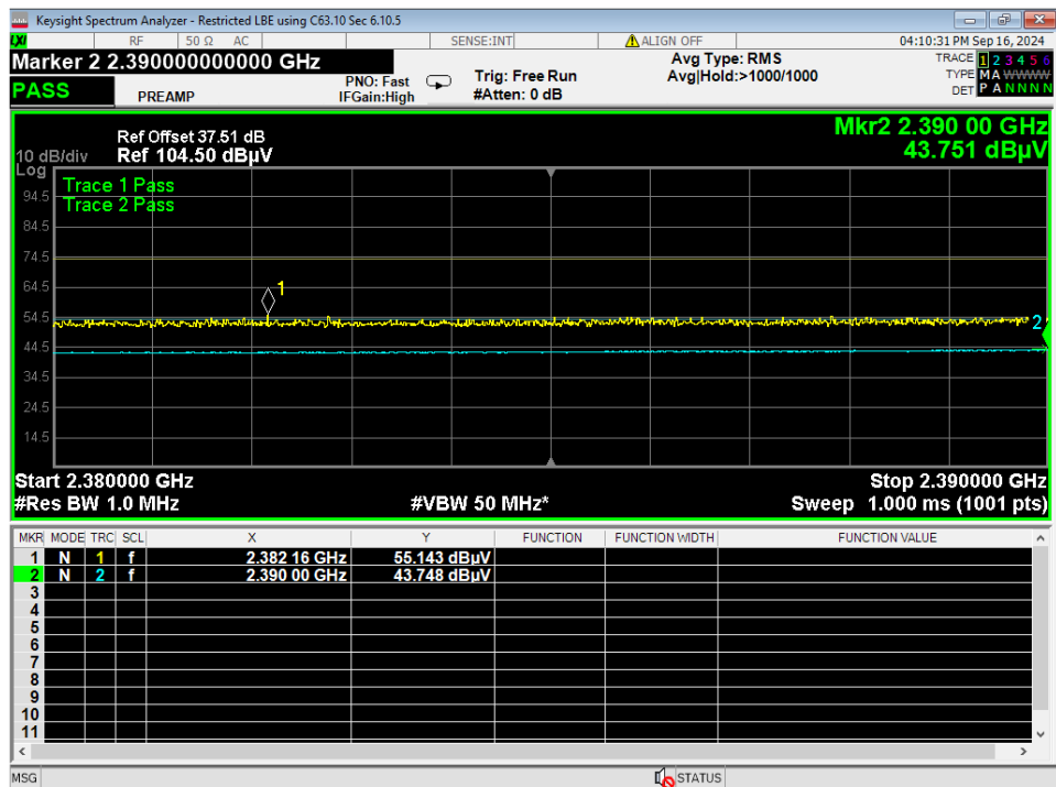
28 LBE Restricted, BLE 2MB
