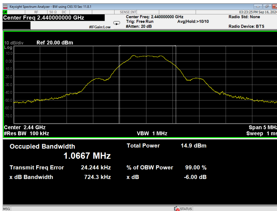
05 6dB Bandwidth, Mid Channel, BLE 1MB
