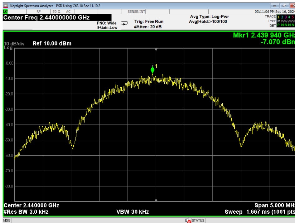
24 PSD, Mid Channel, BLE 2MB
