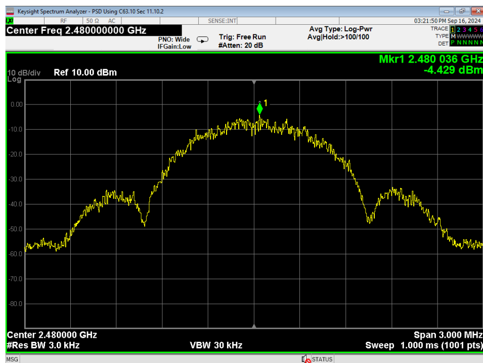
09 PSD, High Channel, BLE 1MB
