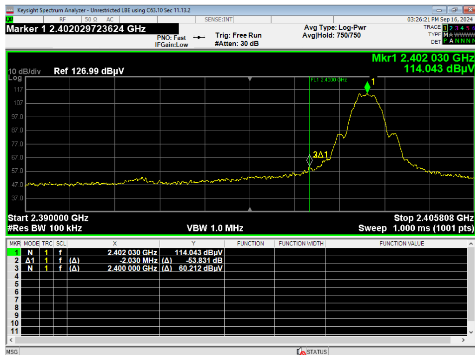
10 LBE Unrestricted, BLE 1MB
