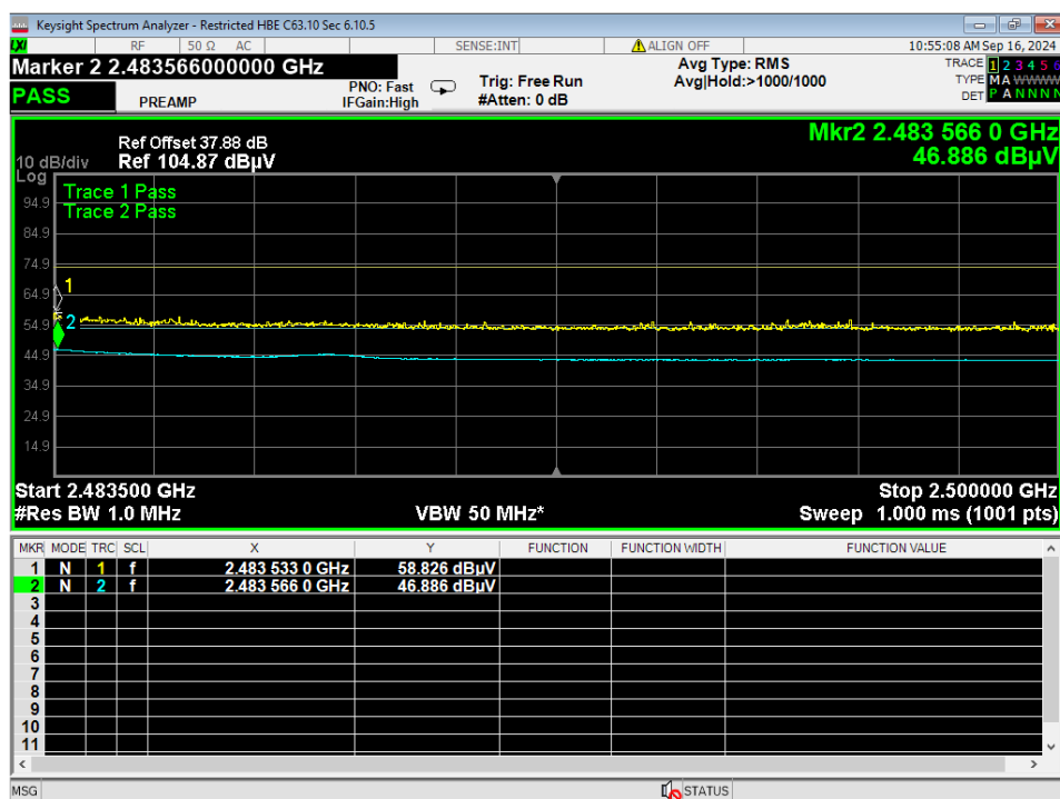
13 HBE Restricted, BLE 1MB
