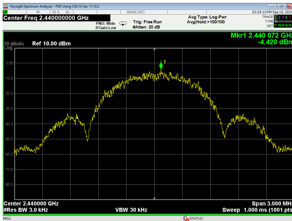
08 PSD, Mid Channel, BLE 1MB
