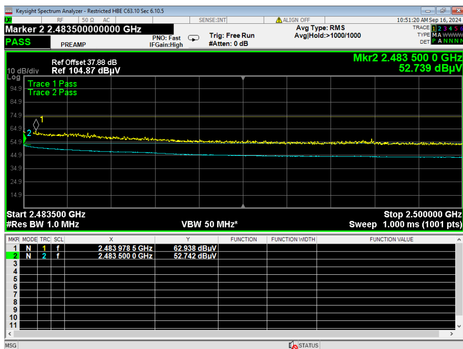
29 HBE Restricted, BLE 2MB
