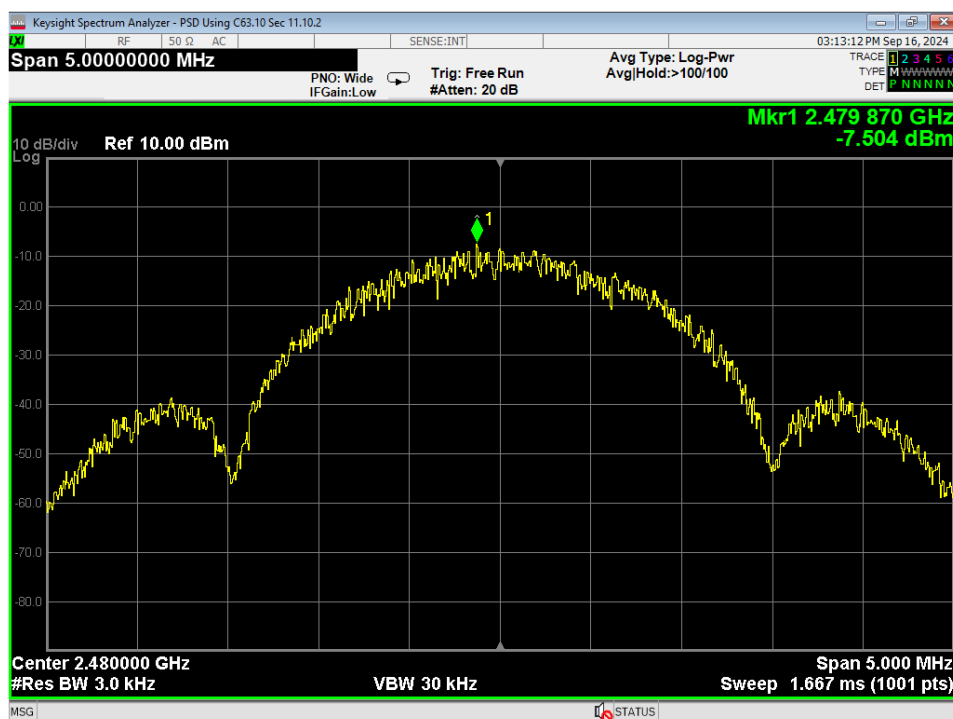
25 PSD, High Channel, BLE 2MB
