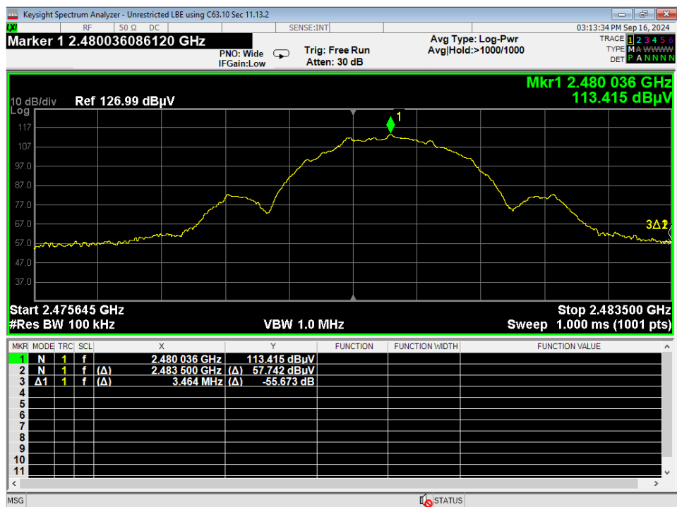
27 HBE Unrestricted, BLE 2MB
