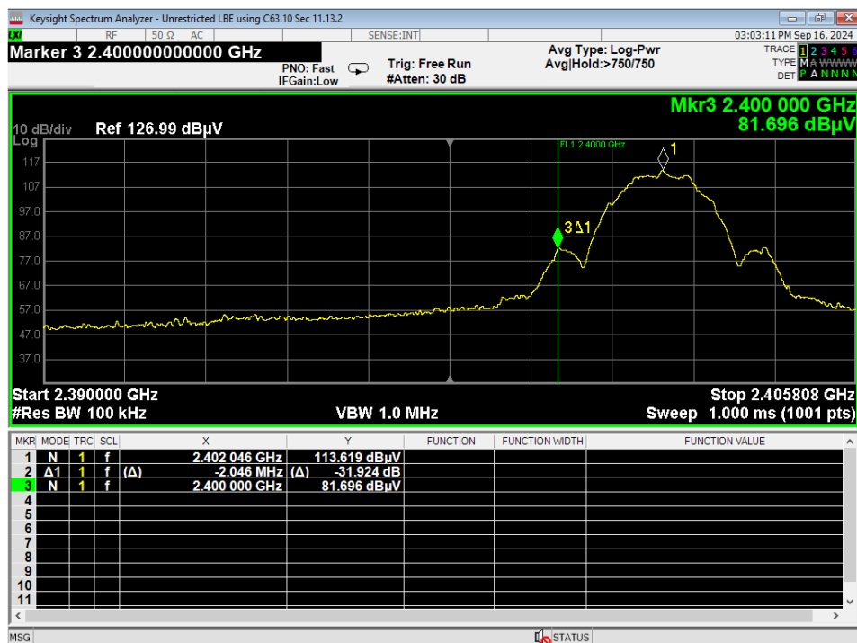
26 LBE Unrestricted, BLE 2MB
