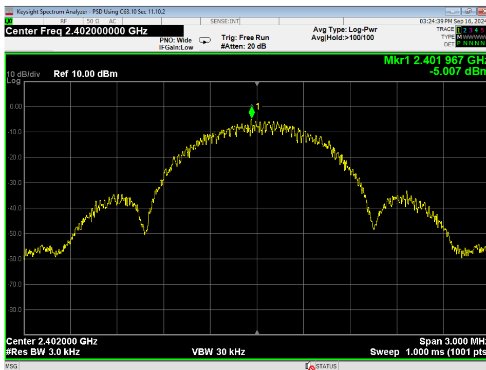
07 PSD, Low Channel, BLE 1MB
