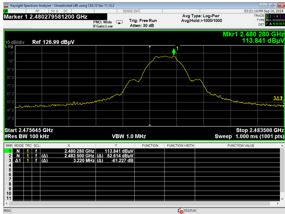
11 HBE Unrestricted, BLE 1MB
