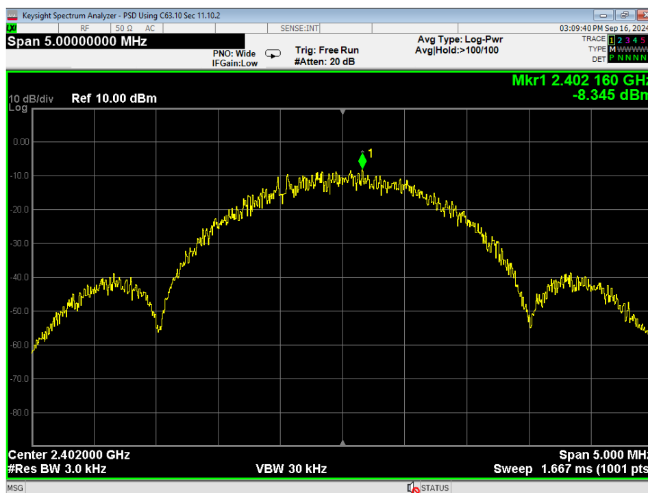
23 PSD, Low Channel, BLE 2MB
