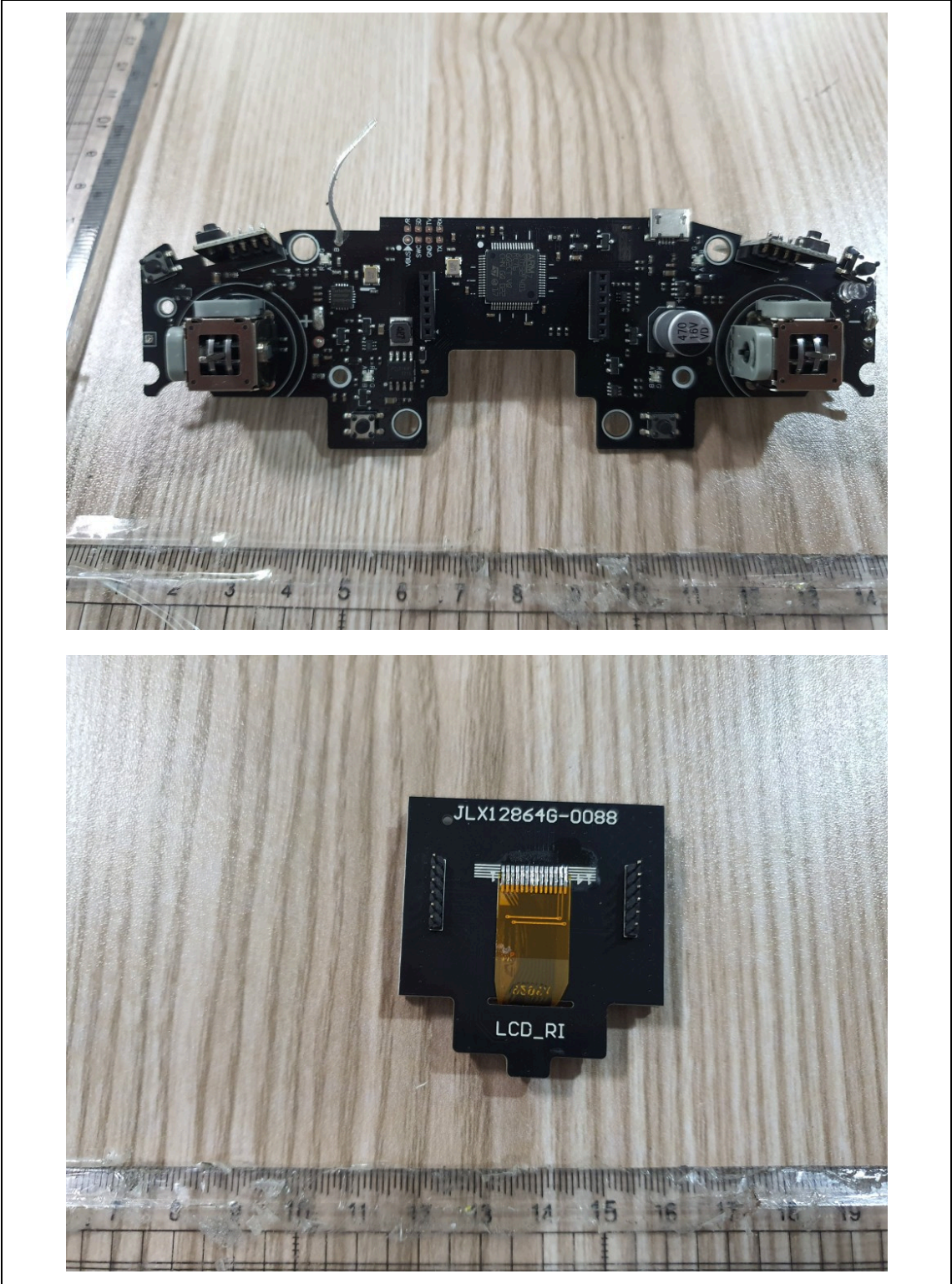
MainBoard-Front
