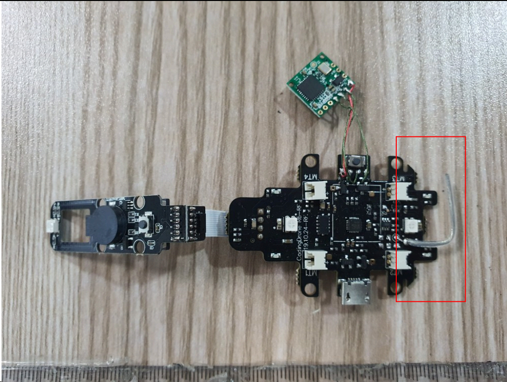
ANTENNA(2.4 GHz)
