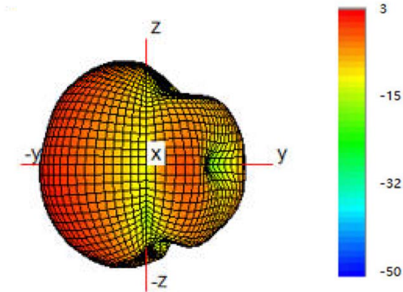
3D 增益模式 3D Gain Pattern (2500 MHz)
