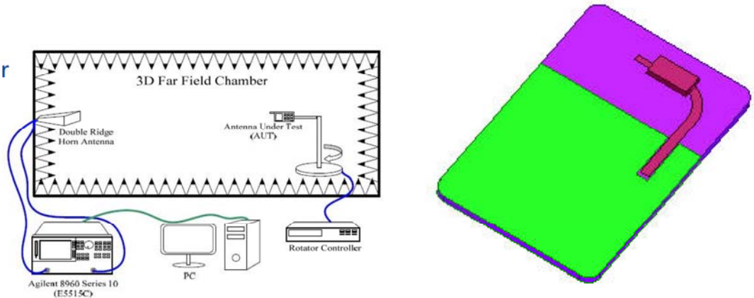
Fig.2 暗室示意图
