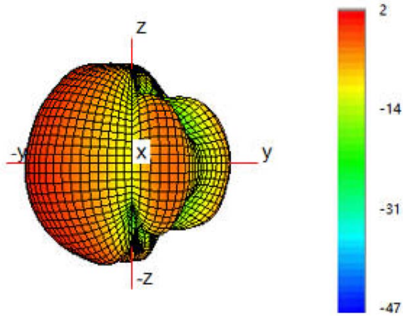
3D 增益模式 3D Gain Pattern (2450 MHz)
