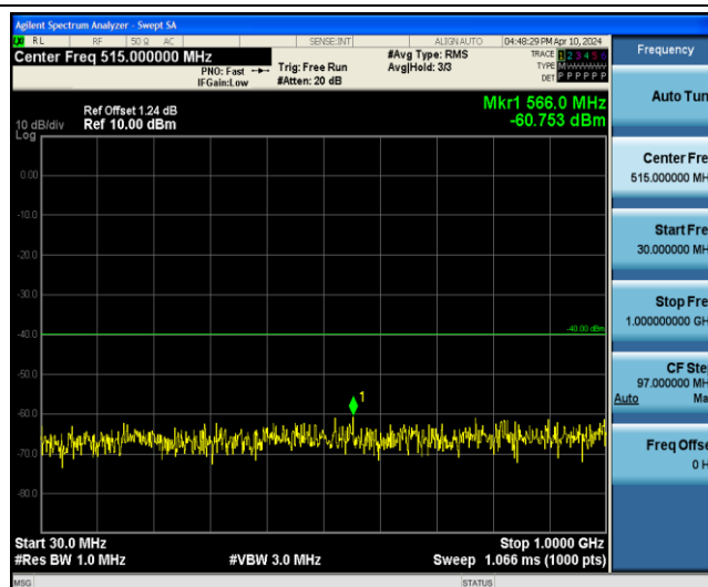
Band40-10MHz-QPSK-39200-1RB#0-Range2:1000~2288MHz
