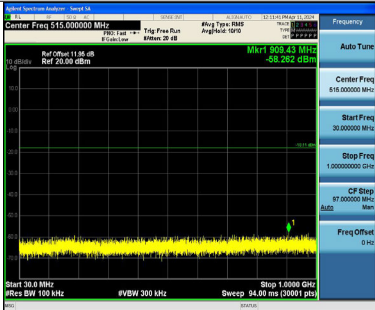
11G-Ant1-2412-30~1000-PASS
