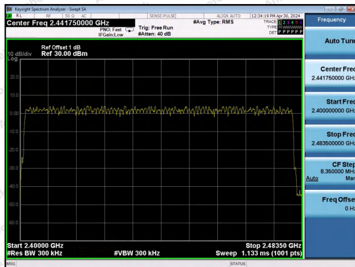
2DH5-Ant0-Hop-PASS
