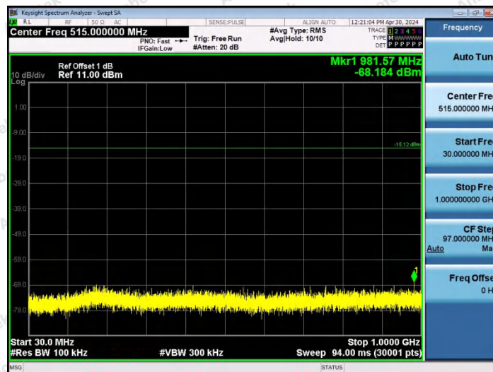
DH5-Ant0-2441-30~1000-PASS
