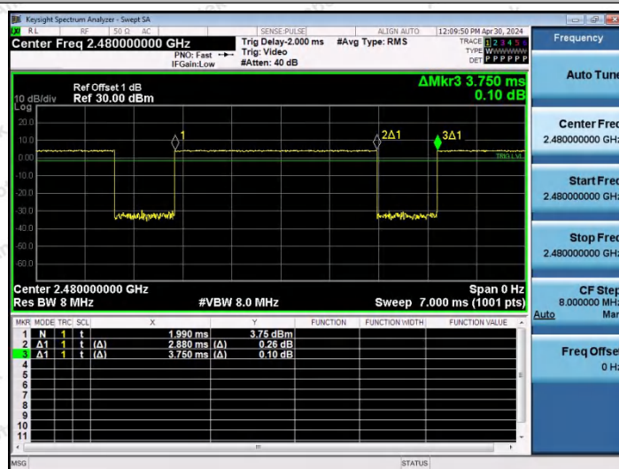
NTVN-2DH5-Ant0-2480
