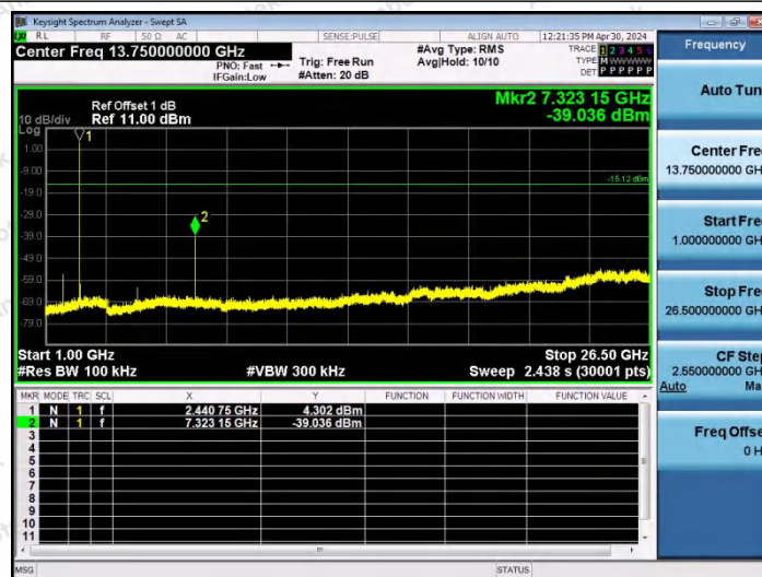
DH5-Ant0-2441-1000~26500-PASS
