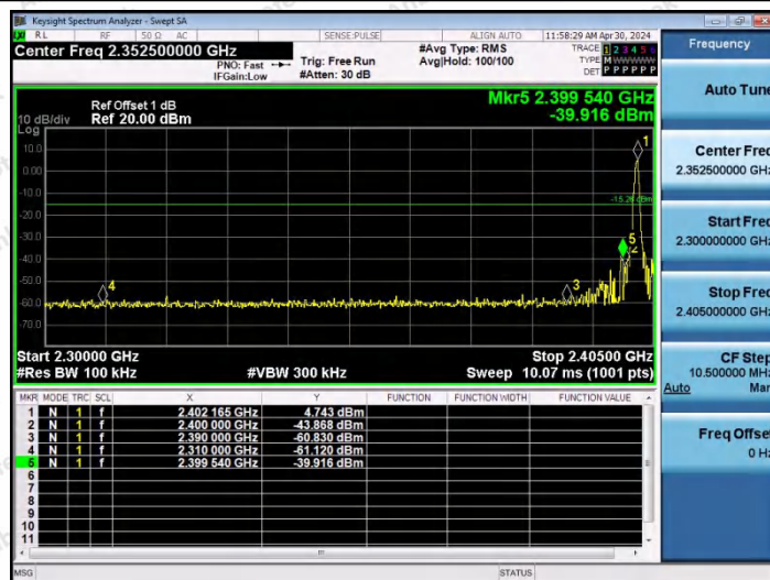
DH5-Ant0-2402-PASS
