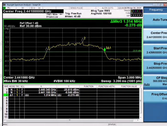
3DH5-Ant0-2441
