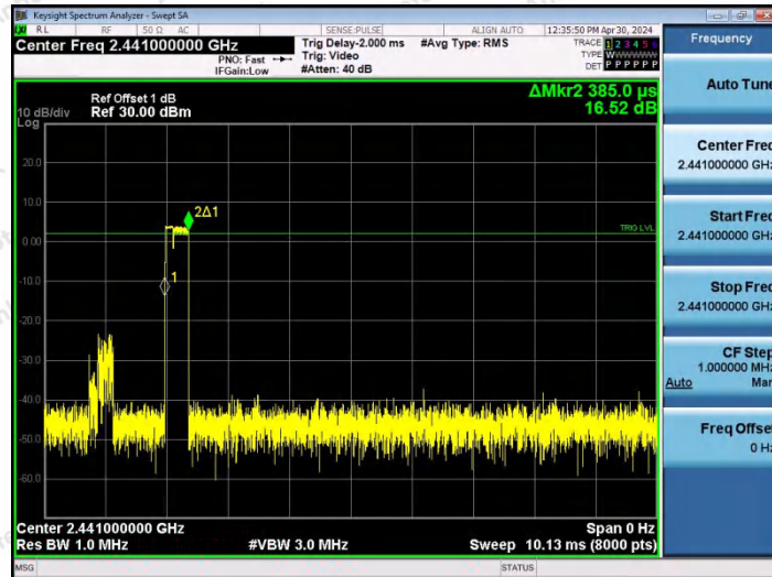
2DH1-Ant0-Hop-PASS
