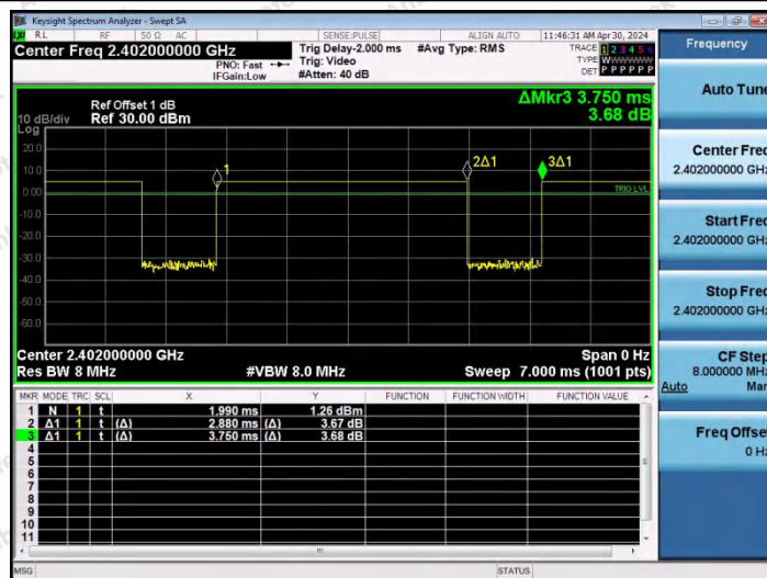
NTNV-DH5-Ant0-2402
