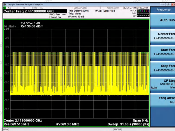
2DH1-Ant0-Hop-PASS
