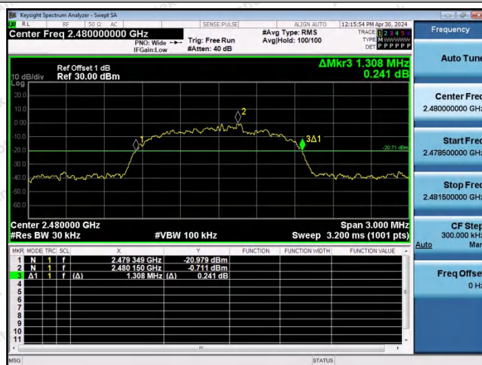
3DH5-Ant0-2480
