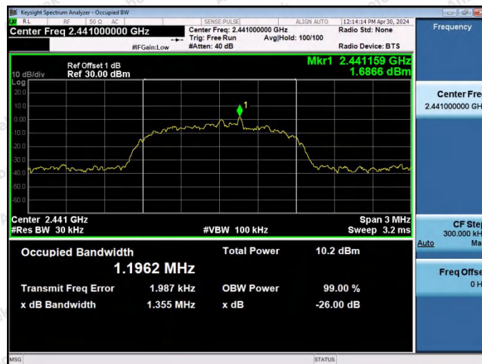
3DH5-Ant0-2441
