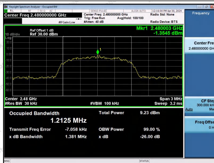
3DH5-Ant0-2480
