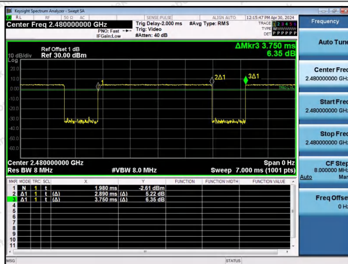
NTVN-3DH5-Ant0-2480
