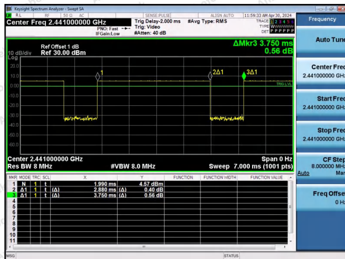
NTNV-DH5-Ant0-2441
