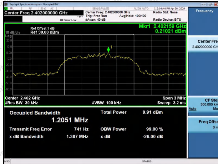
2DH5-Ant0-2402
