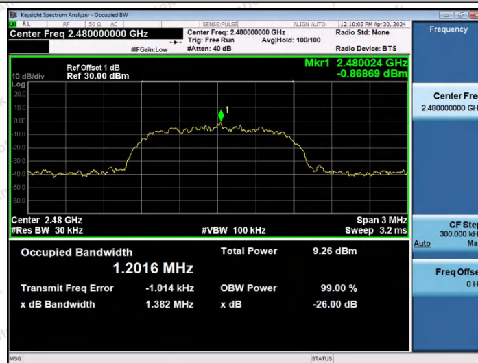
2DH5-Ant0-2480
