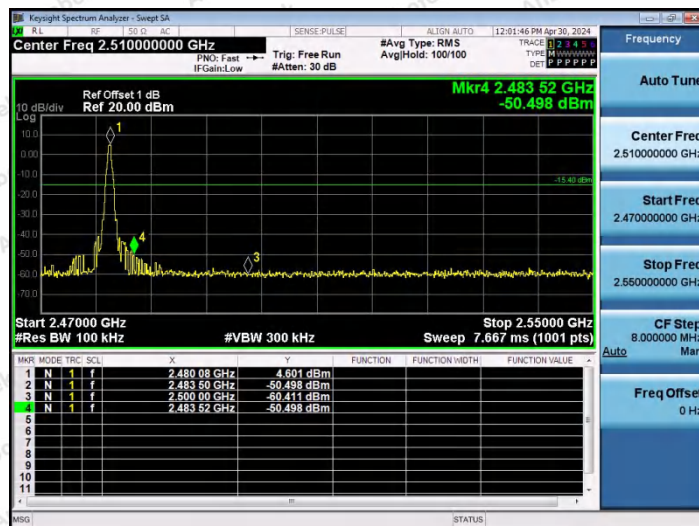
DH5-Ant0-2480-PASS
