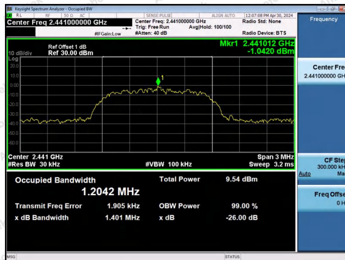
2DH5-Ant0-2441
