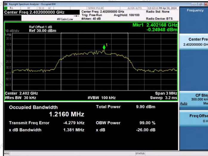
3DH5-Ant0-2402
