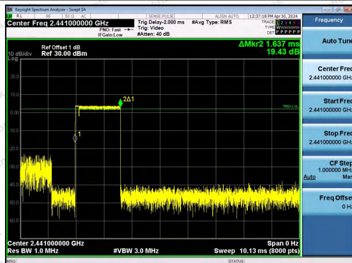
2DH3-Ant0-Hop-PASS
