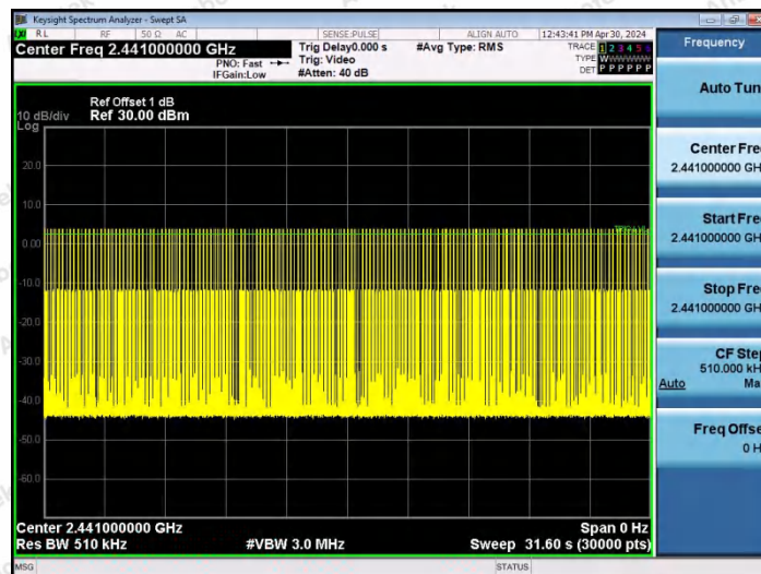
3DH1-Ant0-Hop-PASS
