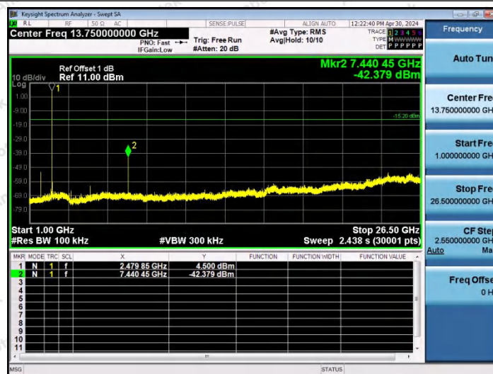
DH5-Ant0-2480-1000~26500-PASS
