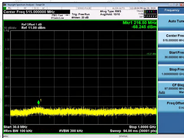
DH5-Ant0-2402-30~1000-PASS
