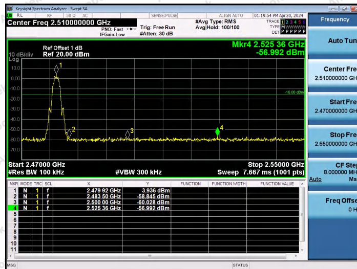
BLE_2M-Ant0-2480-PASS
