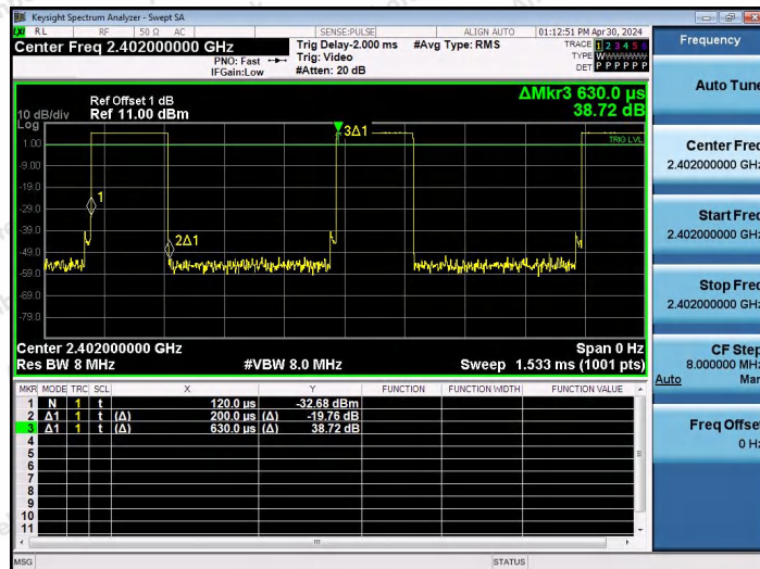
NTNV-BLE_2M-Ant0-2402
