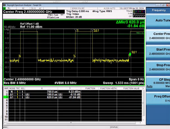
NTNV-BLE_2M-Ant0-2480
