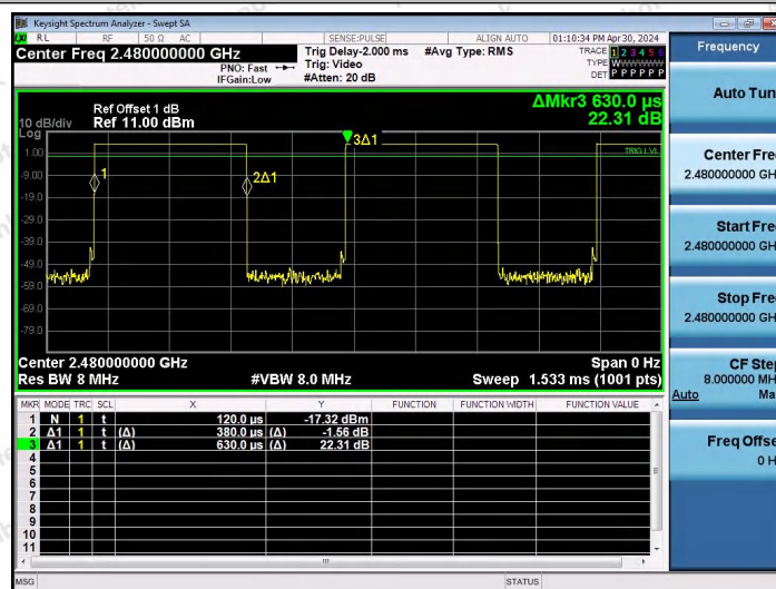
NTNV-BLE_1M-Ant0-2480
