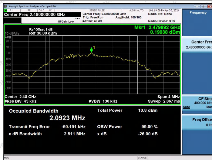
BLE_2M-Ant0-2480
