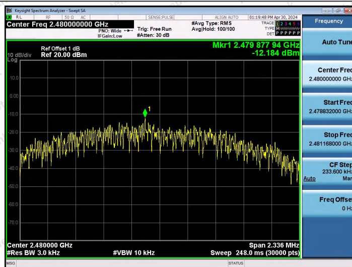
BLE_2M-Ant0-2480-PASS
