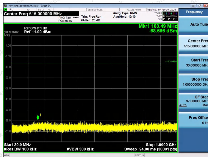
BLE_1M-Ant0-2440-30~1000-PASS
