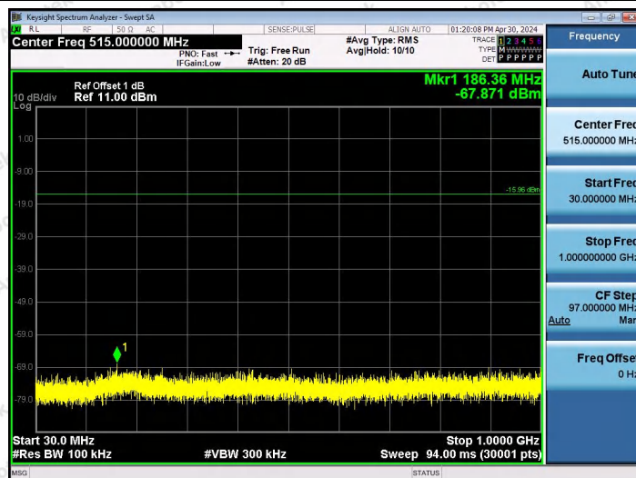
BLE_2M-Ant0-2480-30~1000-PASS
