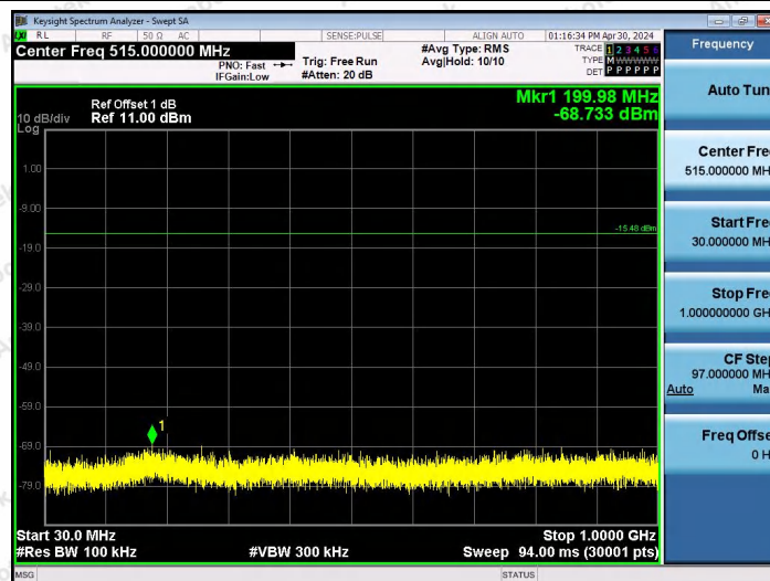
BLE_2M-Ant0-2440-30~1000-PASS
