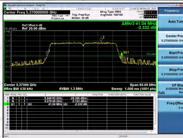
11N40MIMO-Ant0-5270
