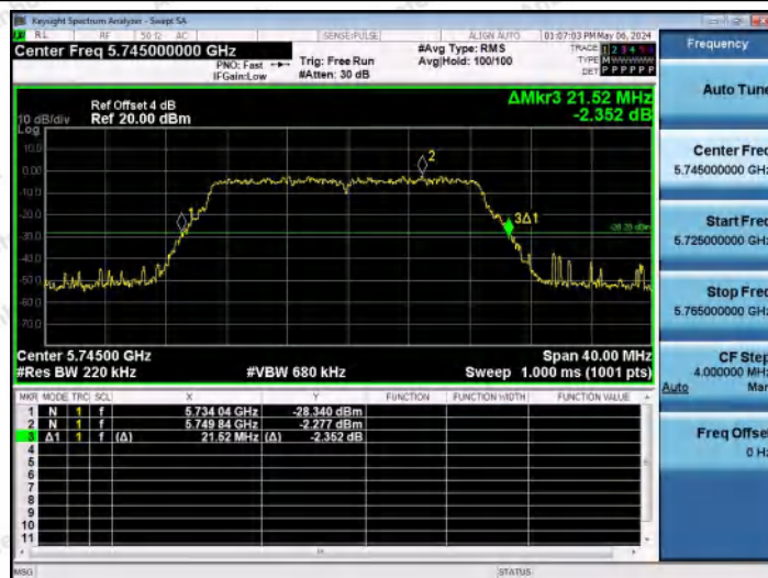
11N20MIMO-Ant0-5745
