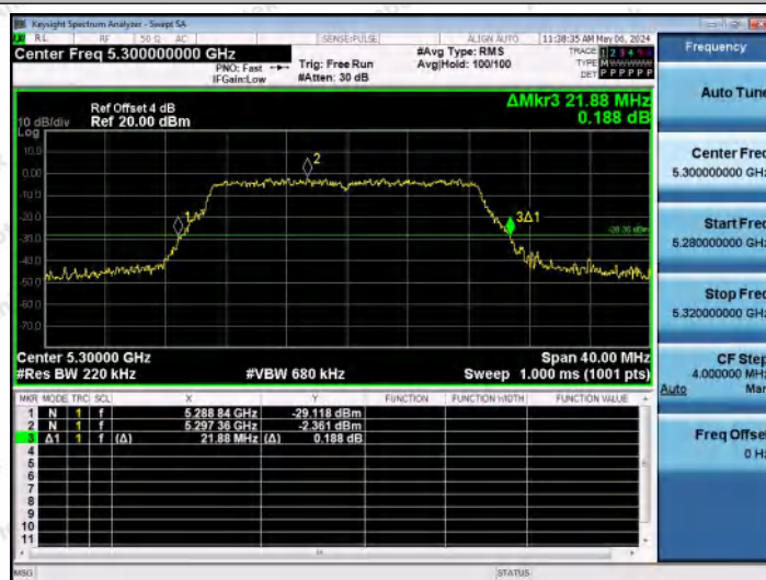
11N20MIMO-Ant0-5300
