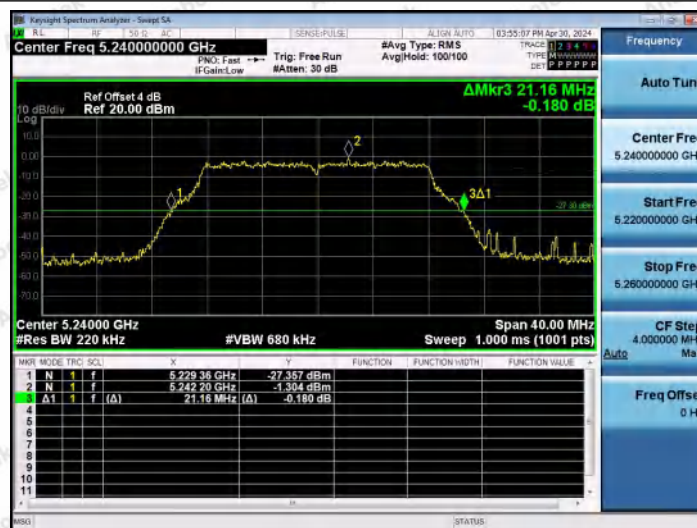
11A-Ant0-5240
