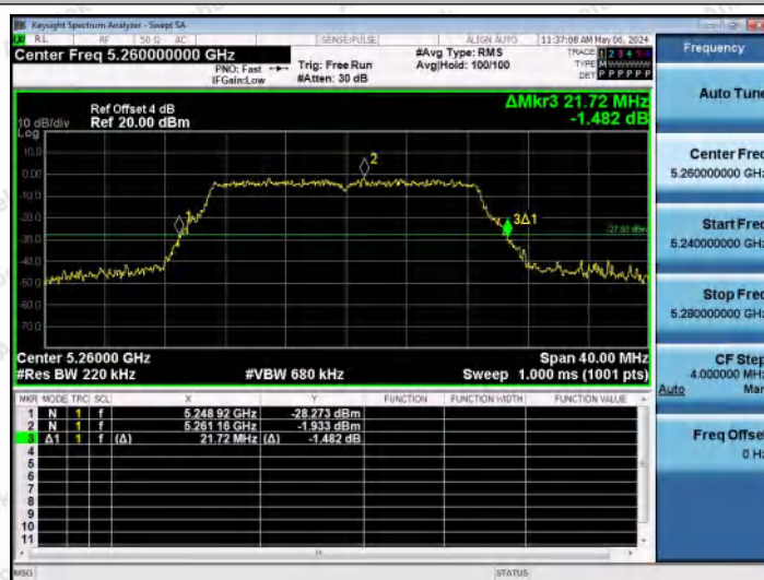
11N20MIMO-Ant1-5260
