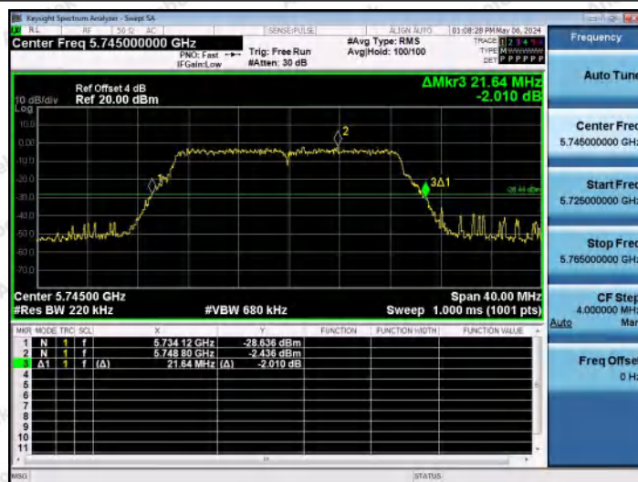
11N20MIMO-Ant1-5745
