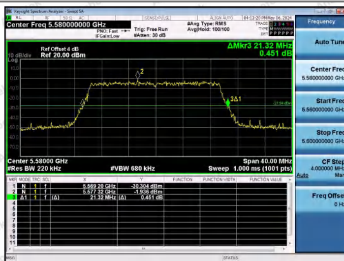
11AX20MIMO-Ant1-5580
