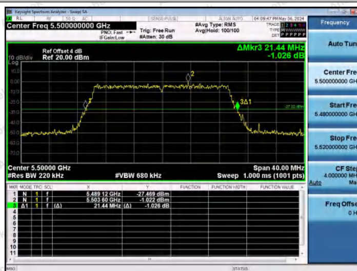
11AX20MIMO-Ant0-5500
