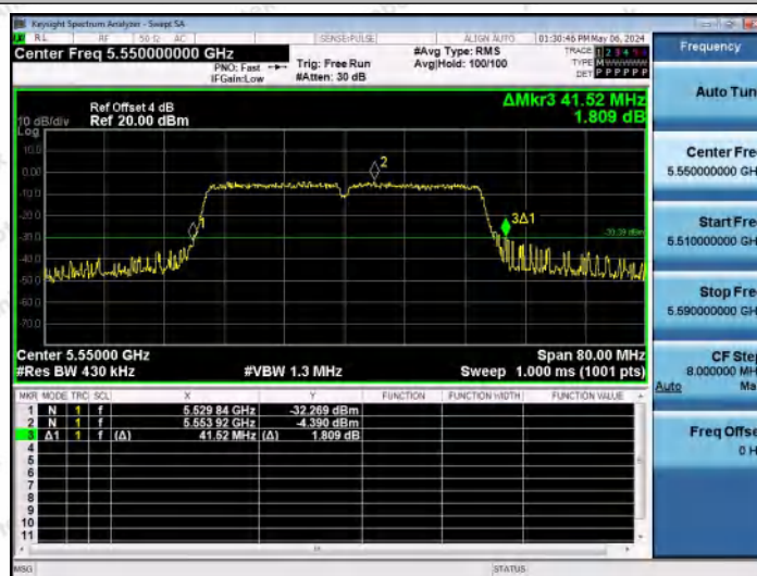
11N40MIMO-Ant1-5550
