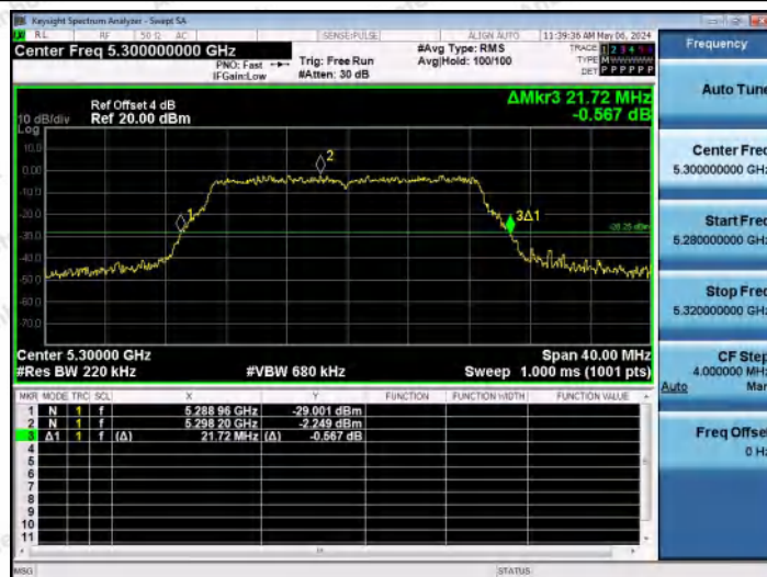
11N20MIMO-Ant1-5300
