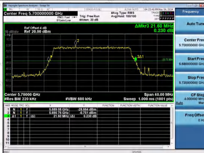
11AX20MIMO-Ant1-5700
