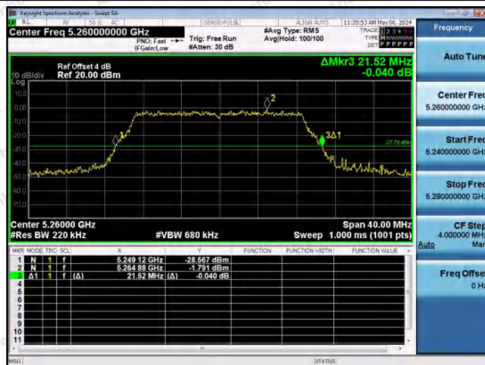
11N20MIMO-Ant0-5260
