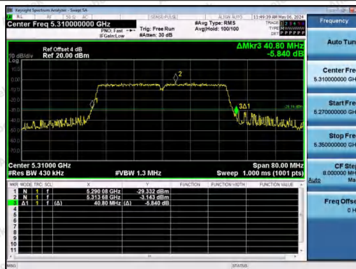
11N40MIMO-Ant1-5310
