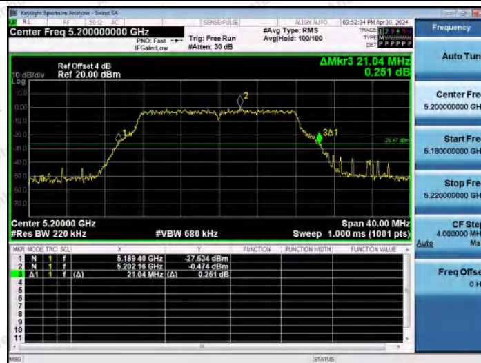
11A-Ant1-5200
