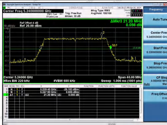
11AX20MIMO-Ant1-5240
