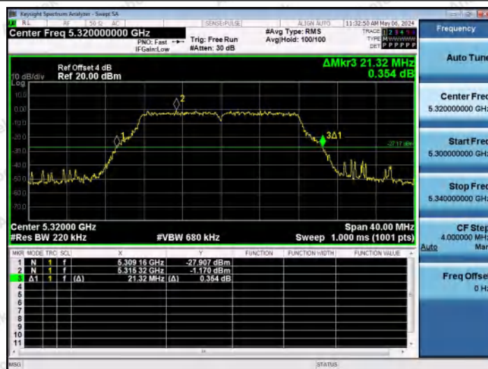
11A-Ant0-5320
