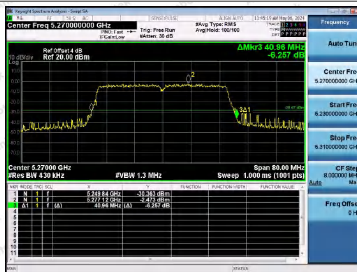
11N40MIMO-Ant1-5270
