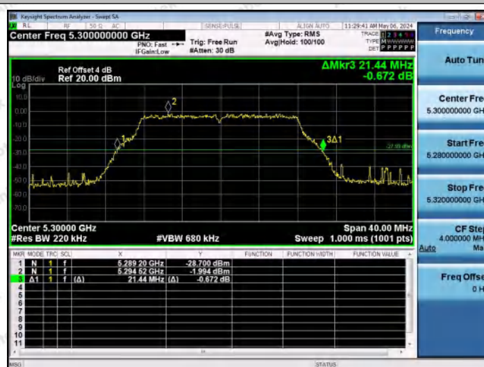
11A-Ant0-5300
