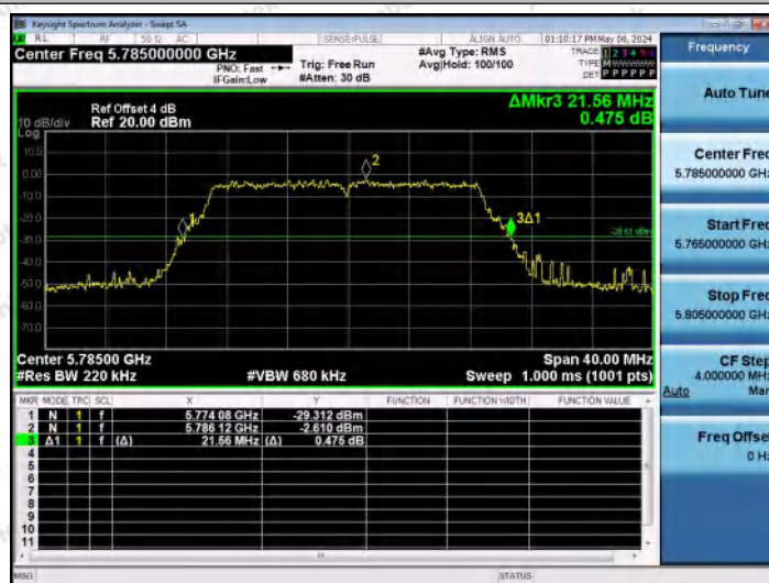
11N20MIMO-Ant0-5785
