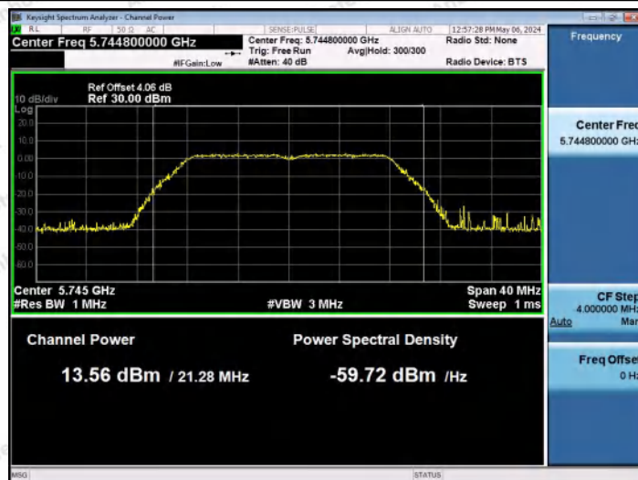
11A-Ant0-5745-PASS
