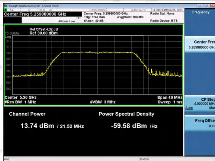
11N20MIMO-Ant0-5260-PASS
