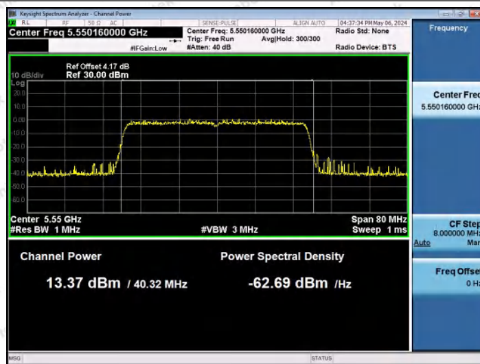
11AX40MIMO-Ant0-5550-PASS
