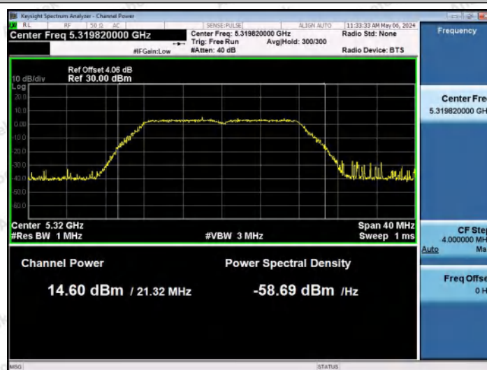
11A-Ant0-5320-PASS
