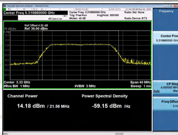
11N20MIMO-Ant0-5320-PASS
