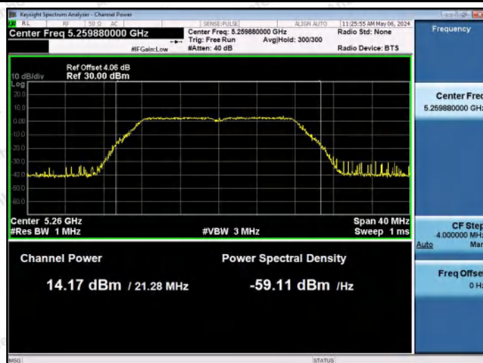
11A-Ant0-5260-PASS
