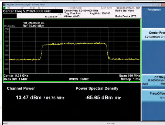
11AX80MIMO-Ant0-5210-PASS
