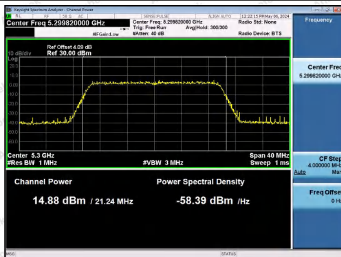
11AX20MIMO-Ant1-5300-PASS
