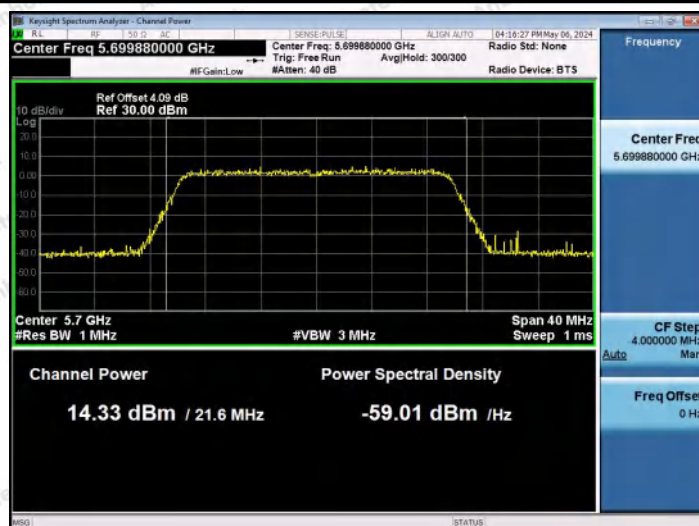
11AX20MIMO-Ant1-5700-PASS
