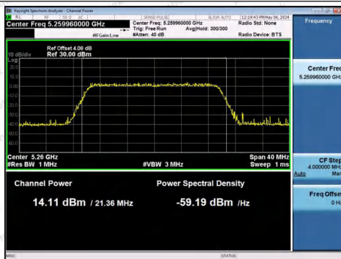
11AX20MIMO-Ant1-5260-PASS
