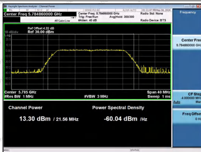
11N20MIMO-Ant0-5785-PASS
