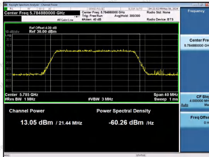
11AX20MIMO-Ant0-5785-PASS
