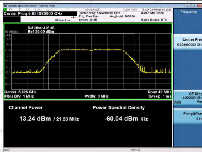
11A-Ant0-5825-PASS
