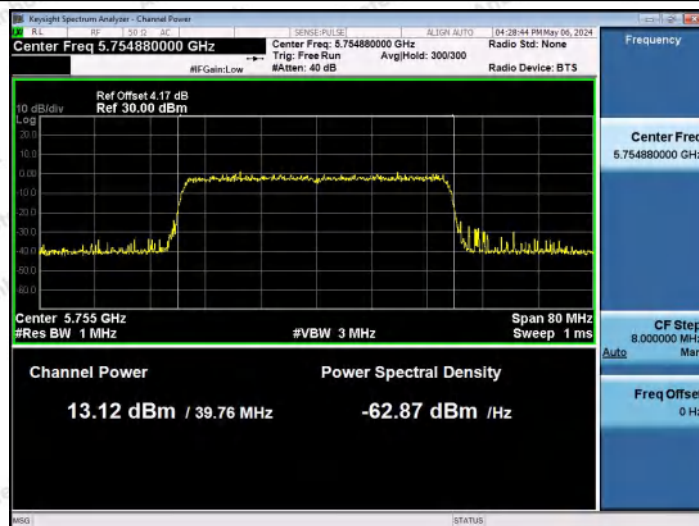
11AX40MIMO-Ant0-5755-PASS
