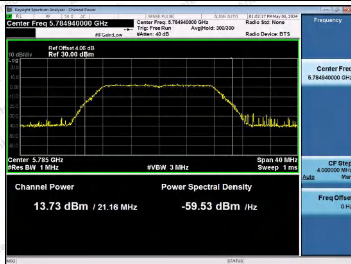
11A-Ant0-5785-PASS
