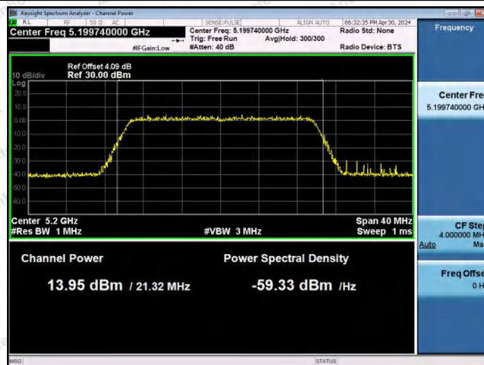
11AX20MIMO-Ant0-5200-PASS
