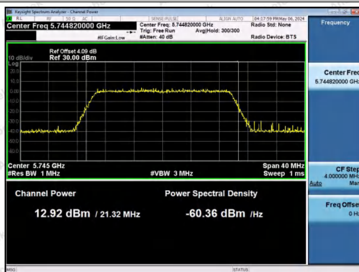
11AX20MIMO-Ant0-5745-PASS
