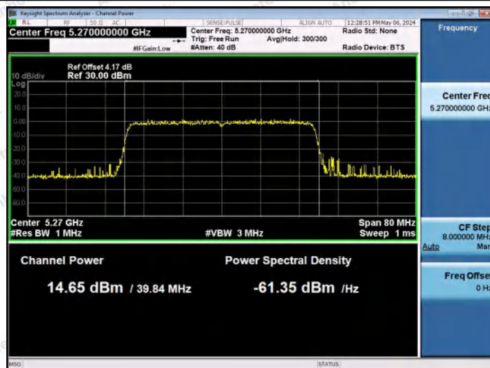
11AX40MIMO-Ant1-5270-PASS
