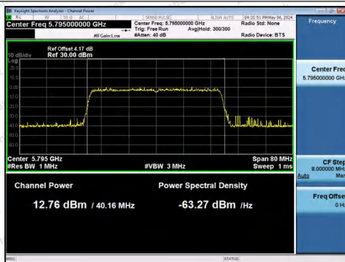
11AX40MIMO-Ant0-5795-PASS
