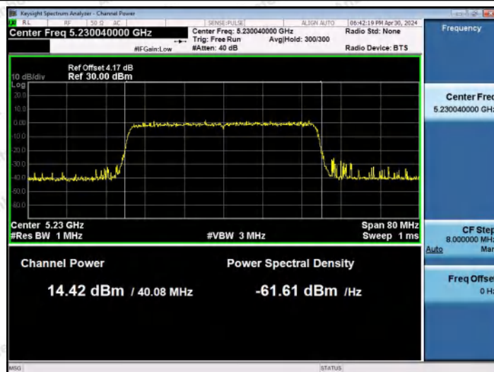
11AX40MIMO-Ant0-5230-PASS
