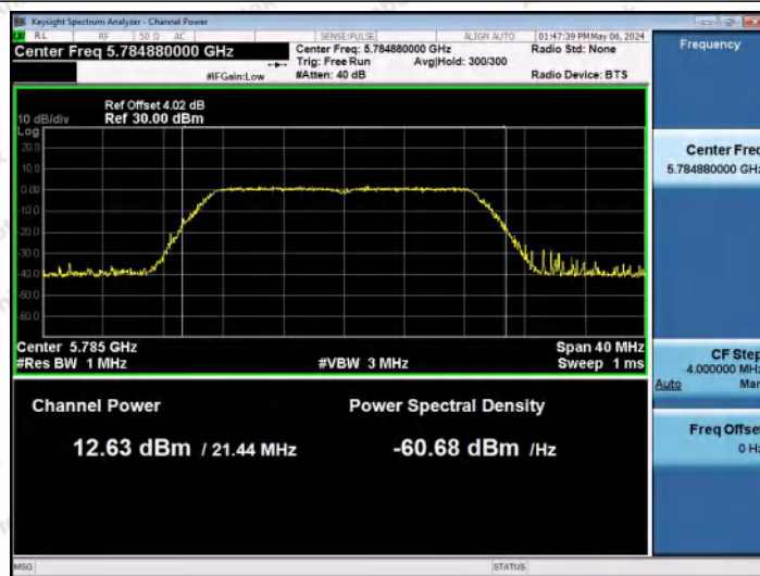
11AC20MIMO-Ant0-5785-PASS
