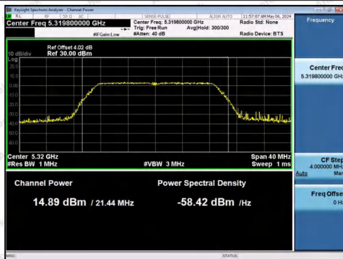
11AC20MIMO-Ant0-5320-PASS
