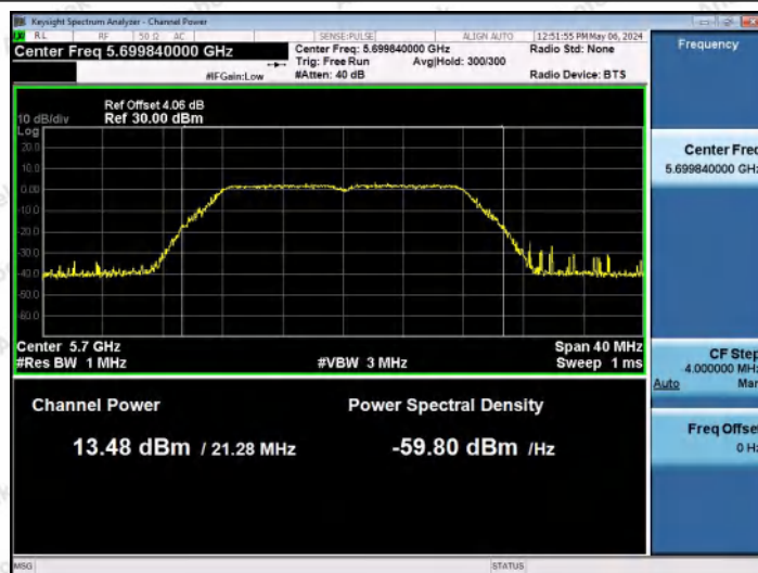
11A-Ant0-5700-PASS
