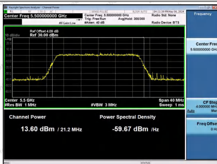
11AX20MIMO-Ant1-5500-PASS
