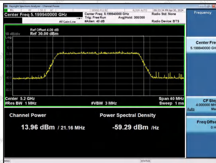
11AX20MIMO-Ant1-5200-PASS
