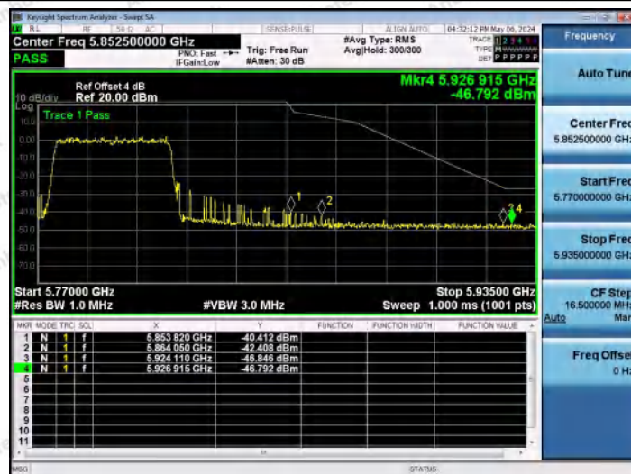
11AX40MIMO-Ant0-5795-PASS
