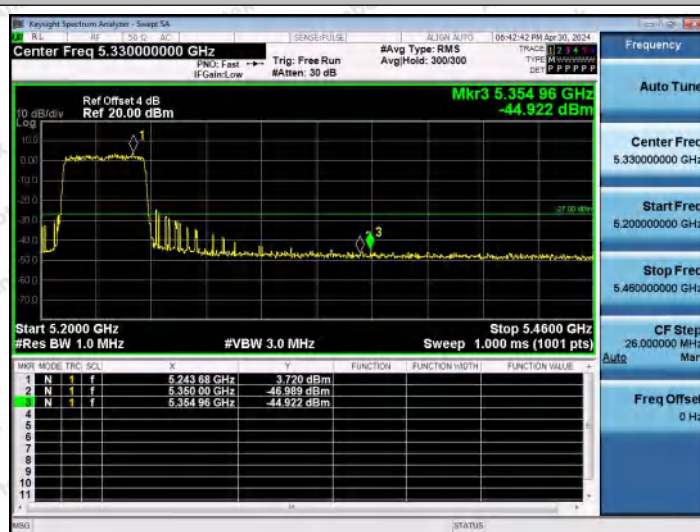
11AX40MIMO-Ant0-5230-PASS
