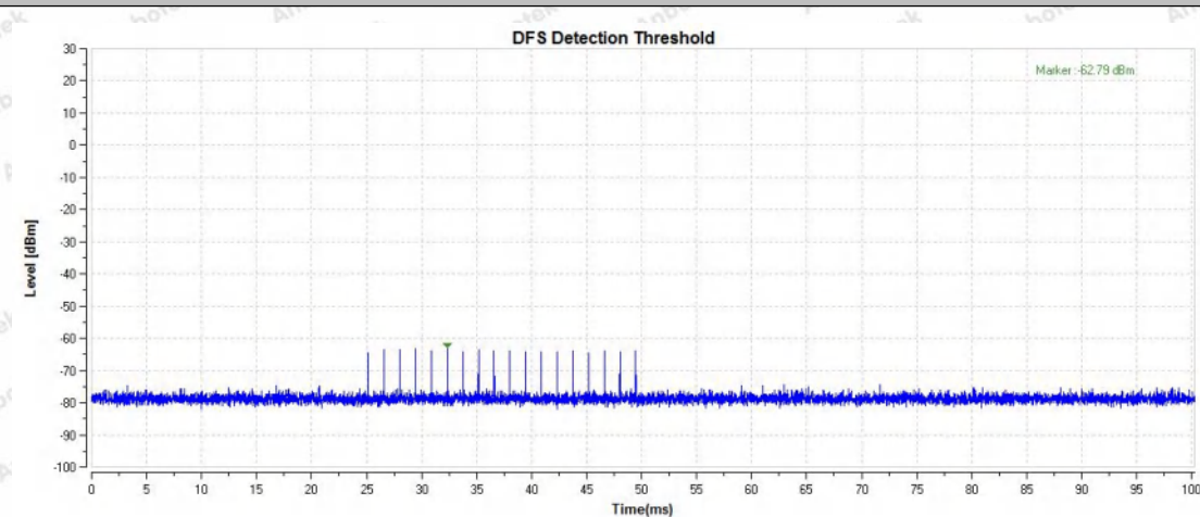
11AC80SISO_5290_Type0
