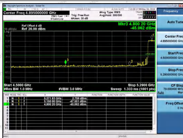
11AX40MIMO-Ant1-5270-PASS
