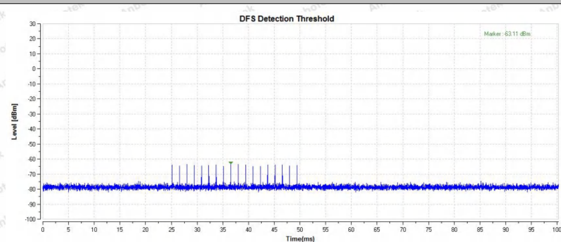
11AC80SISO_5610_Type0
