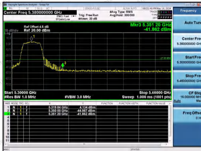
11AC20MIMO-Ant0-5320-PASS
