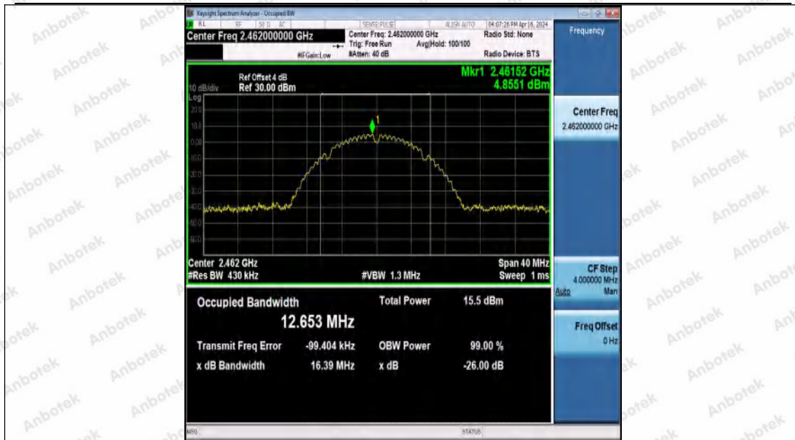
11B-Ant0-2462
