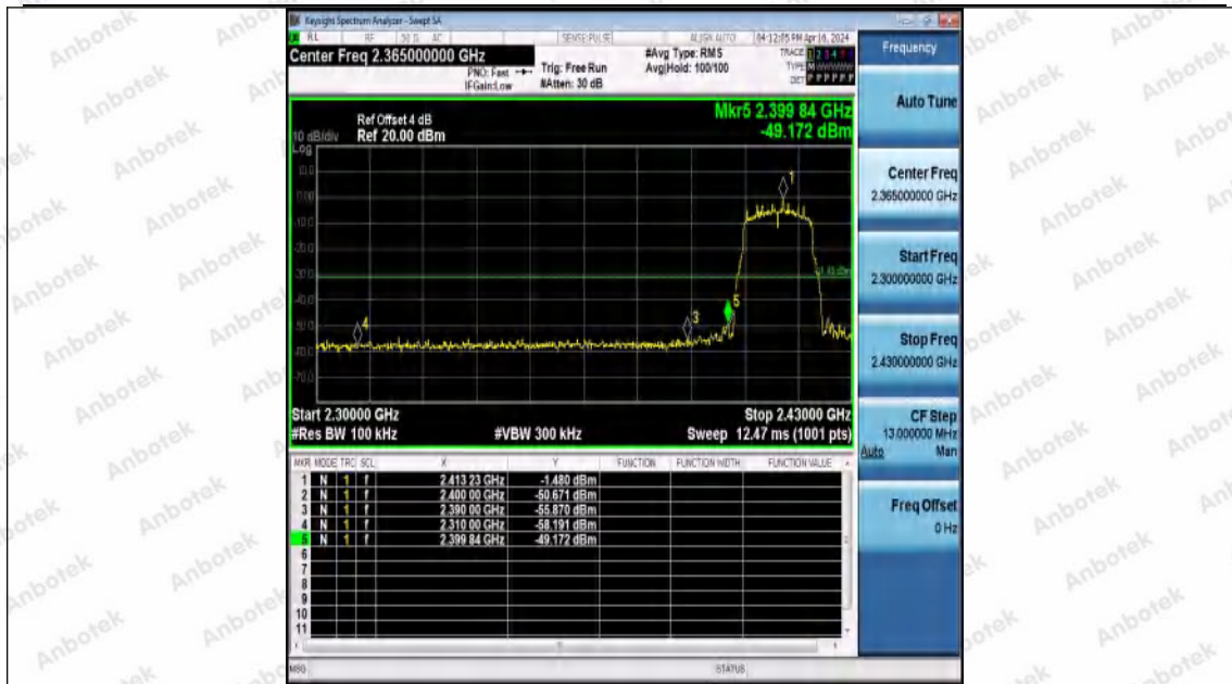
11G-Ant0-2412-PASS
