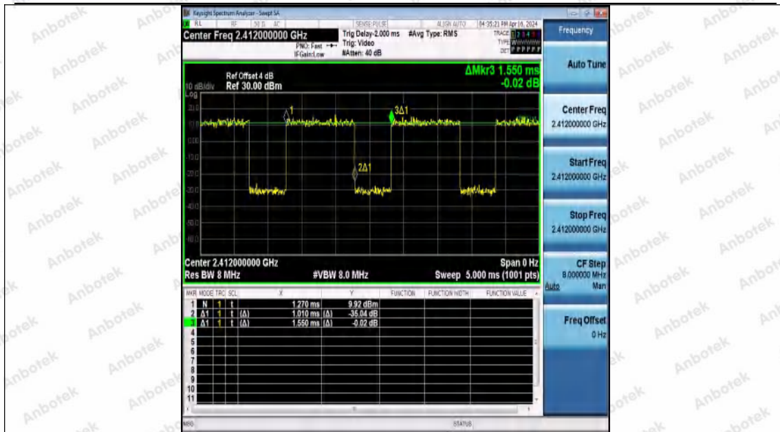
NTNV-11AX20MIMO-Ant0-2412
