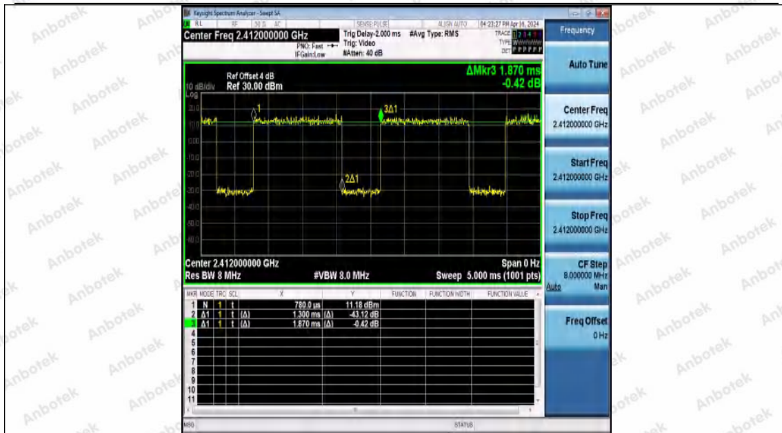
NTNV-11N20MIMO-Ant0-2412
