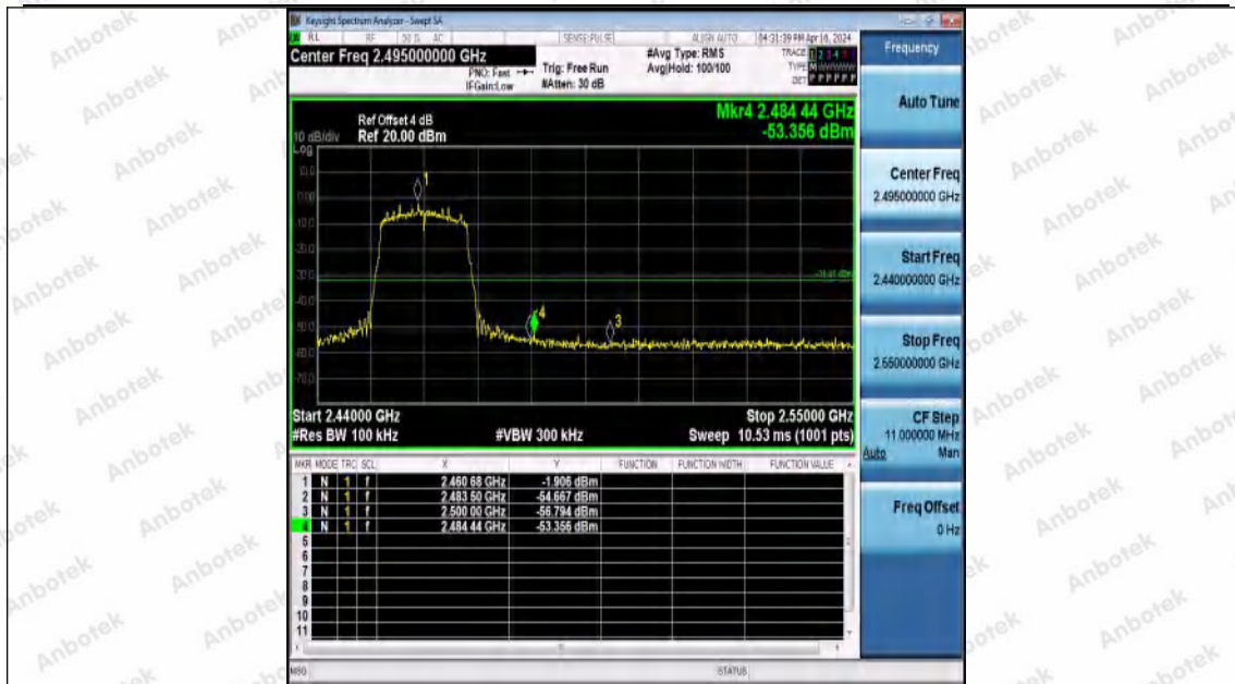
11N20MIMO-Ant0-2462-PASS
