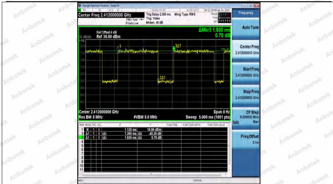
NTNV-11G-Ant0-2412
