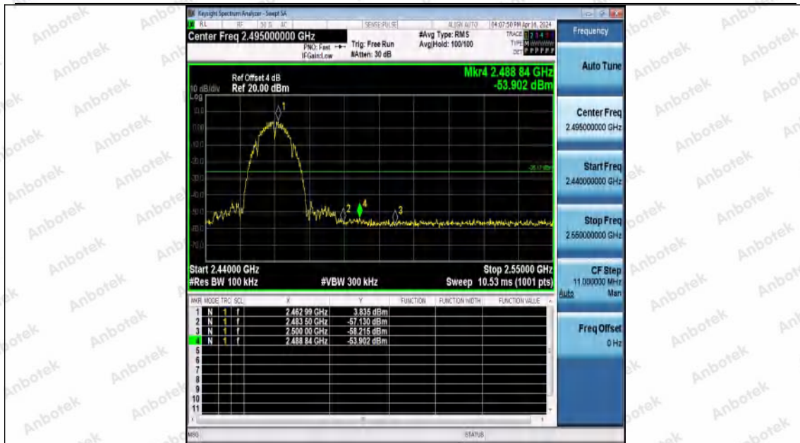
11B-Ant0-2462-PASS
