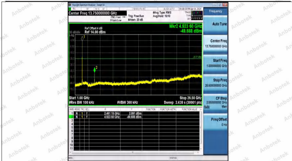
11B-Ant0-2462-1000~26500-PASS
