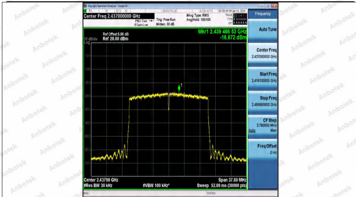
11AX20MIMO-Ant0-2437-PASS
