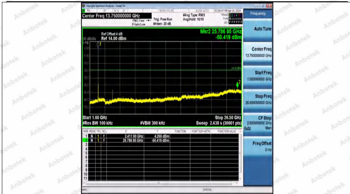
11B-Ant0-2412-1000~26500-PASS
