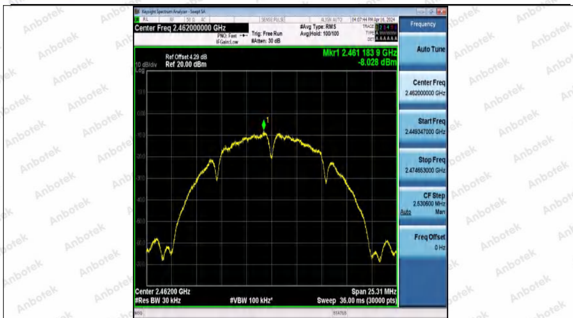
11B-Ant0-2462-PASS
