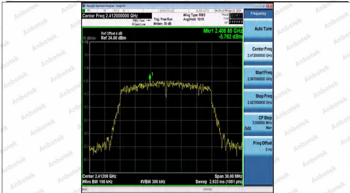
11N20MIMO-Ant0-2412-0-Reference-PASS
