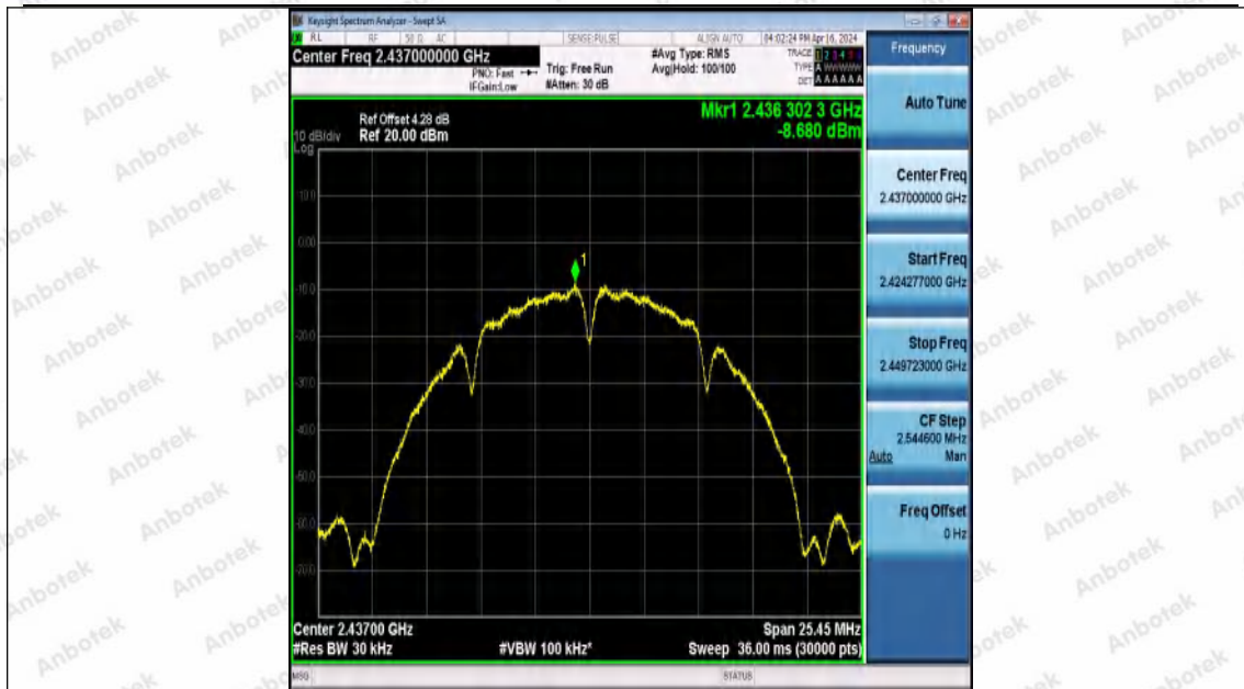
11B-Ant0-2437-PASS
