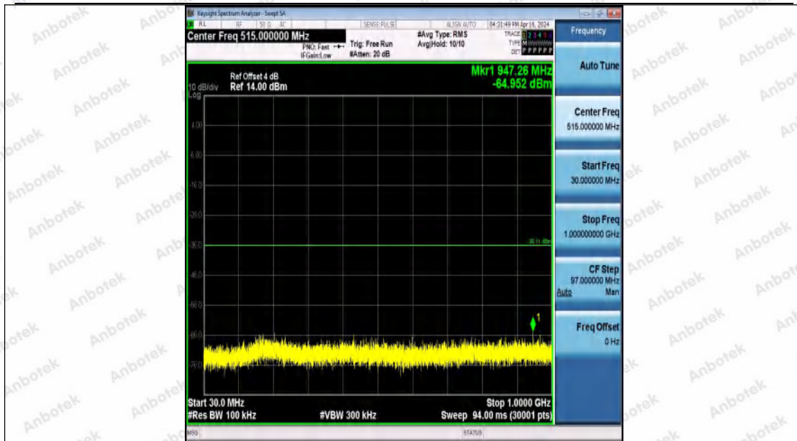
11N20MIMO-Ant0-2462-30~1000-PASS
