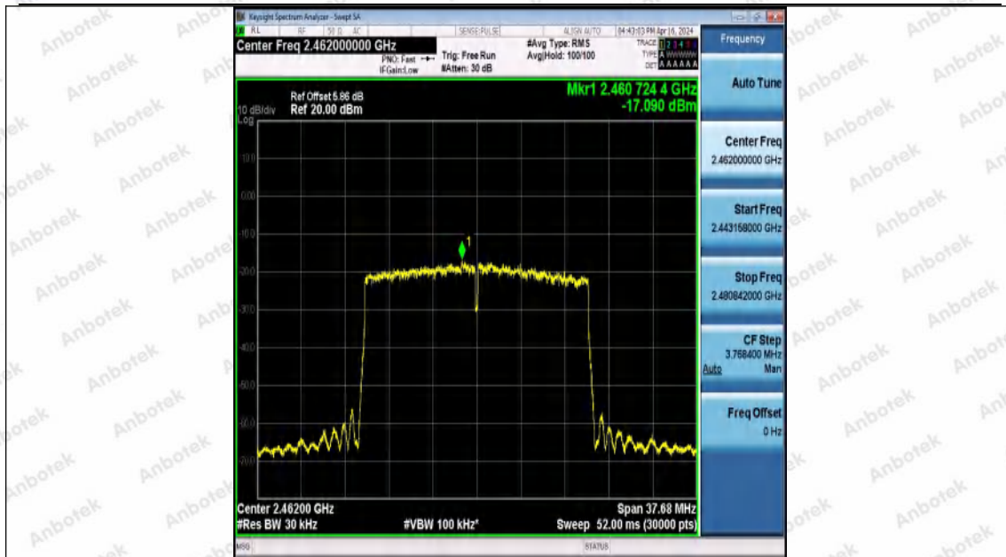
11AX20MIMO-Ant0-2462-PASS
