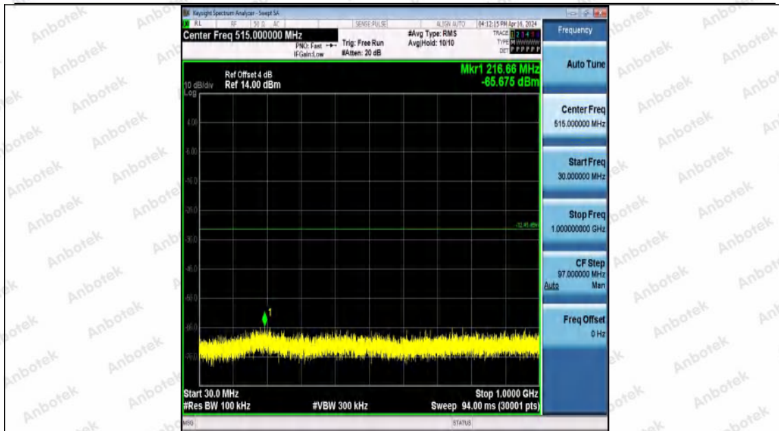
11G-Ant0-2412-30~1000-PASS
