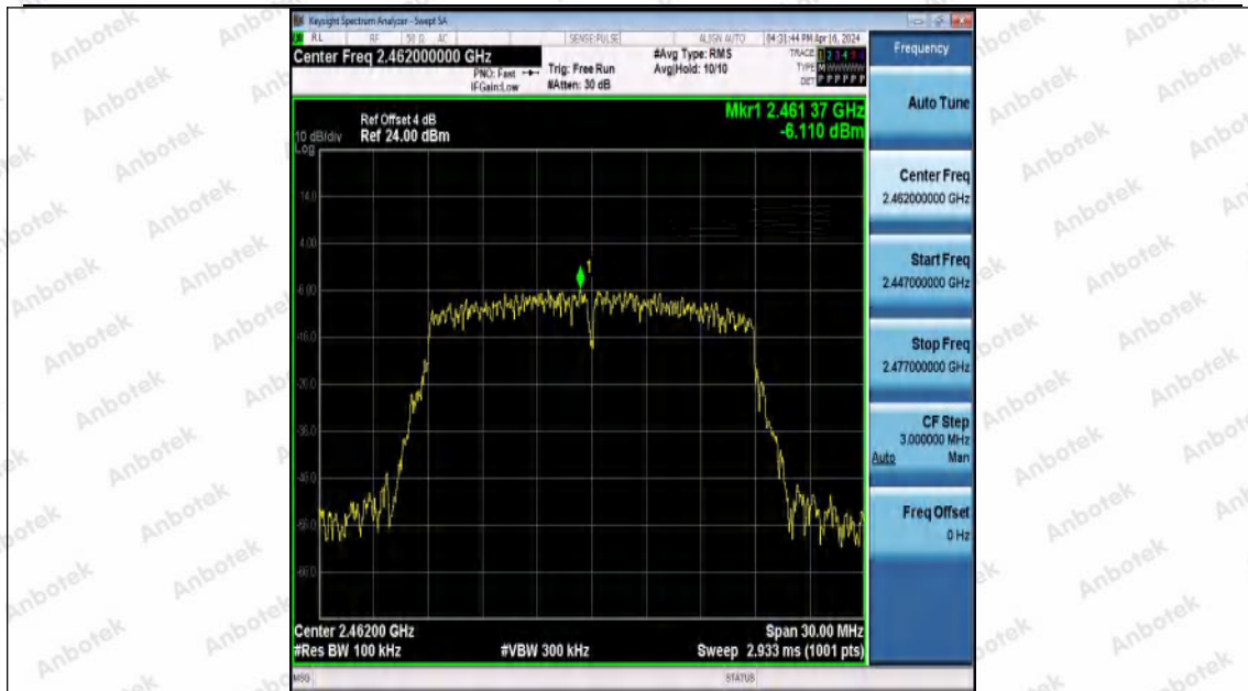
11N20MIMO-Ant0-2462-0-Reference-PASS
