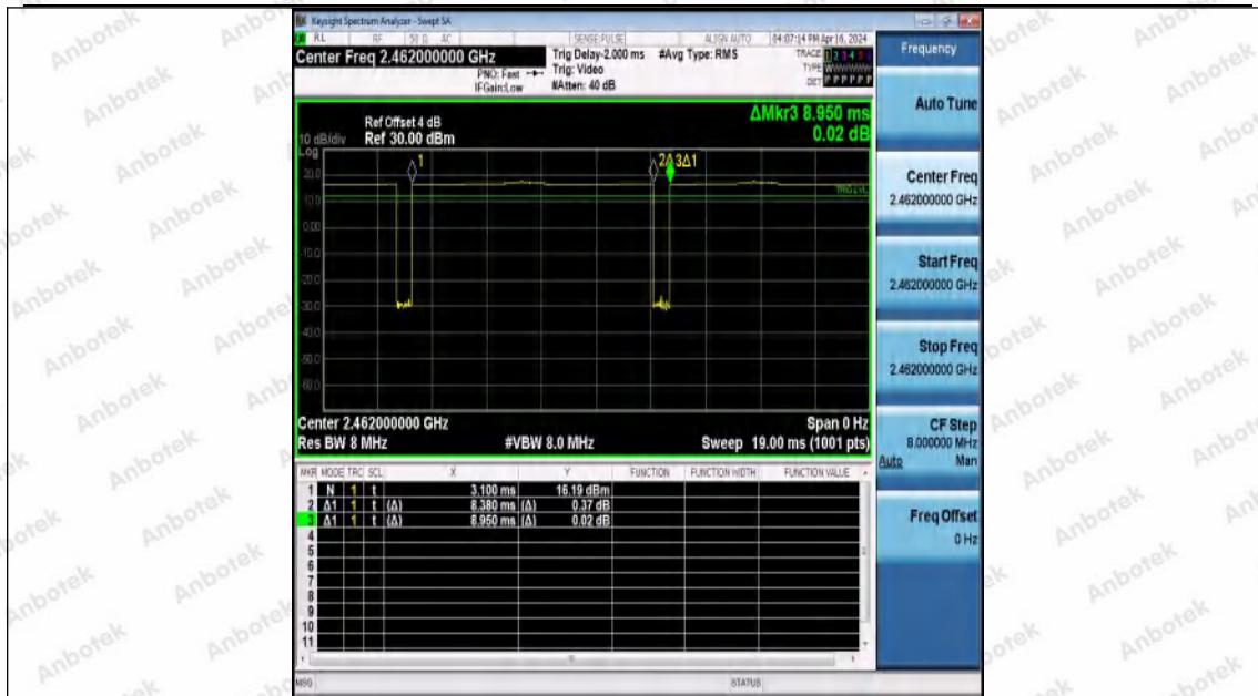
NTNV-11B-Ant0-2462
