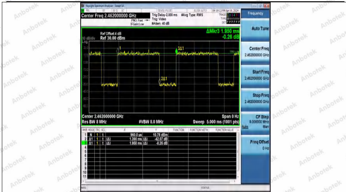
NTNV-11G-Ant0-2462
