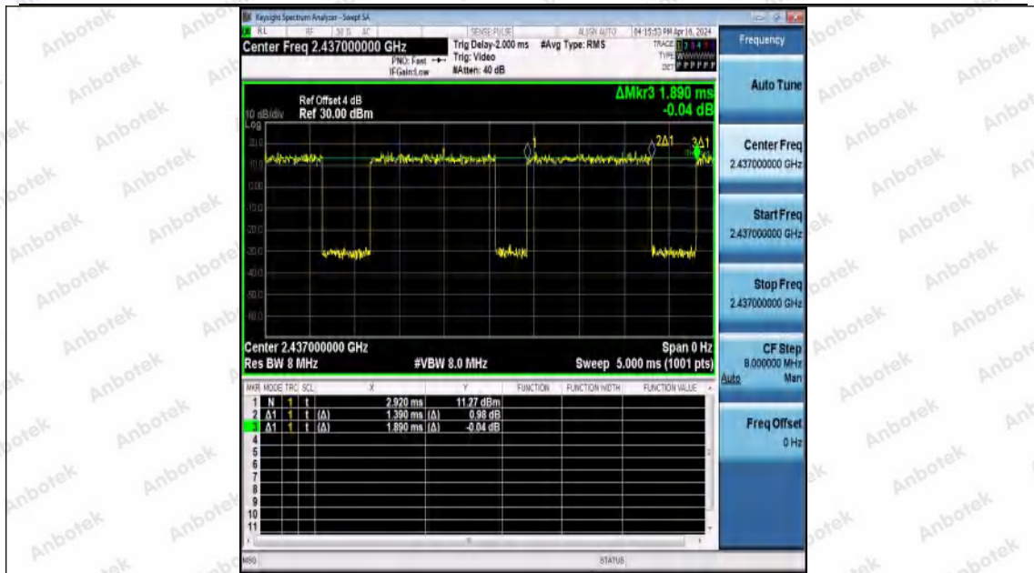
NTNV-11G-Ant0-2437
