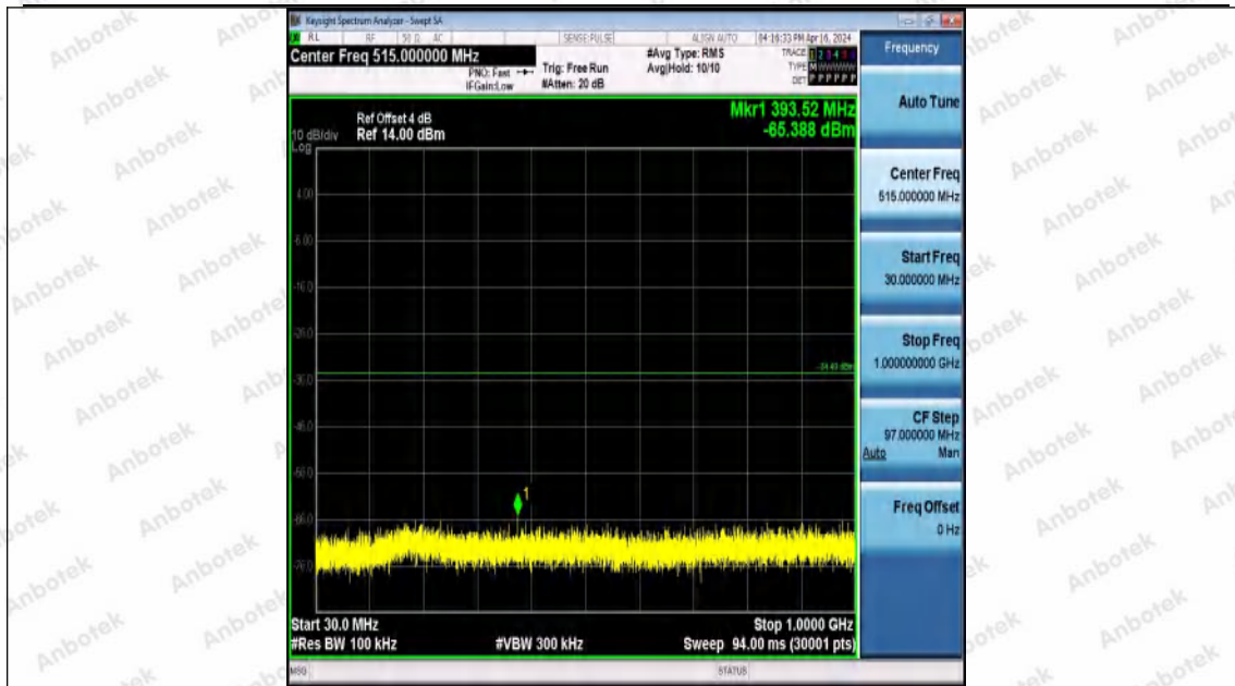
11G-Ant0-2437-30~1000-PASS
