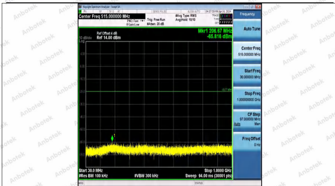
11B-Ant0-2462-30~1000-PASS
