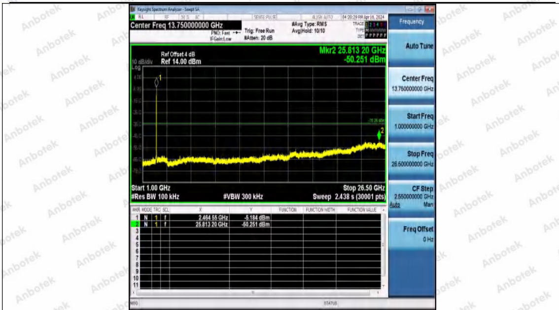
11G-Ant0-2462-1000~26500-PASS
