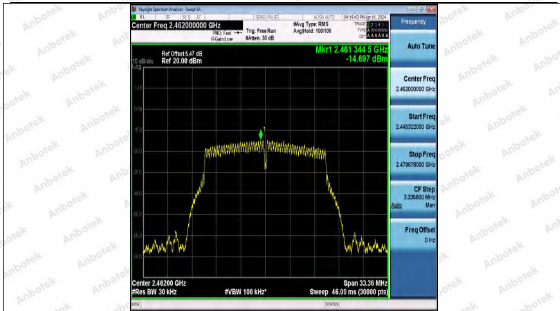
11G-Ant0-2462-PASS
