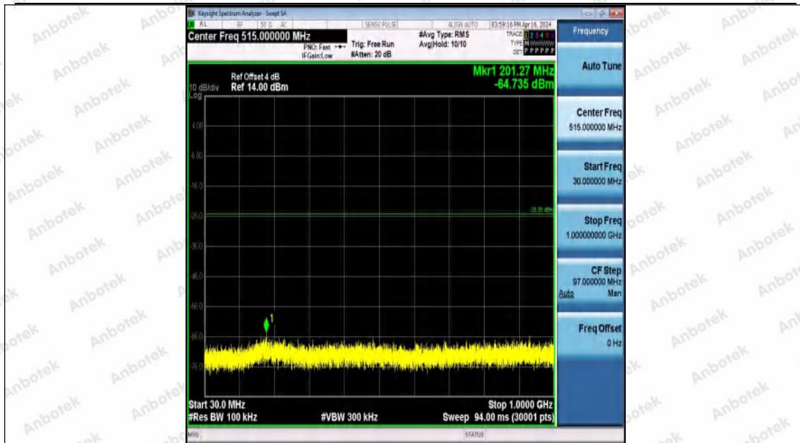
11B-Ant0-2412-30~1000-PASS
