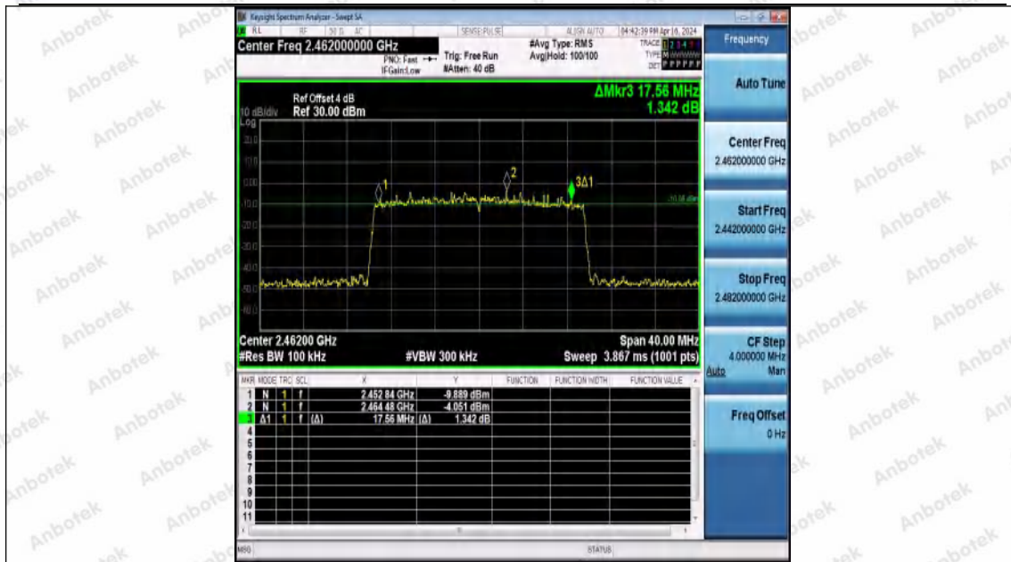
11AX20MIMO-Ant0-2462-PASS
