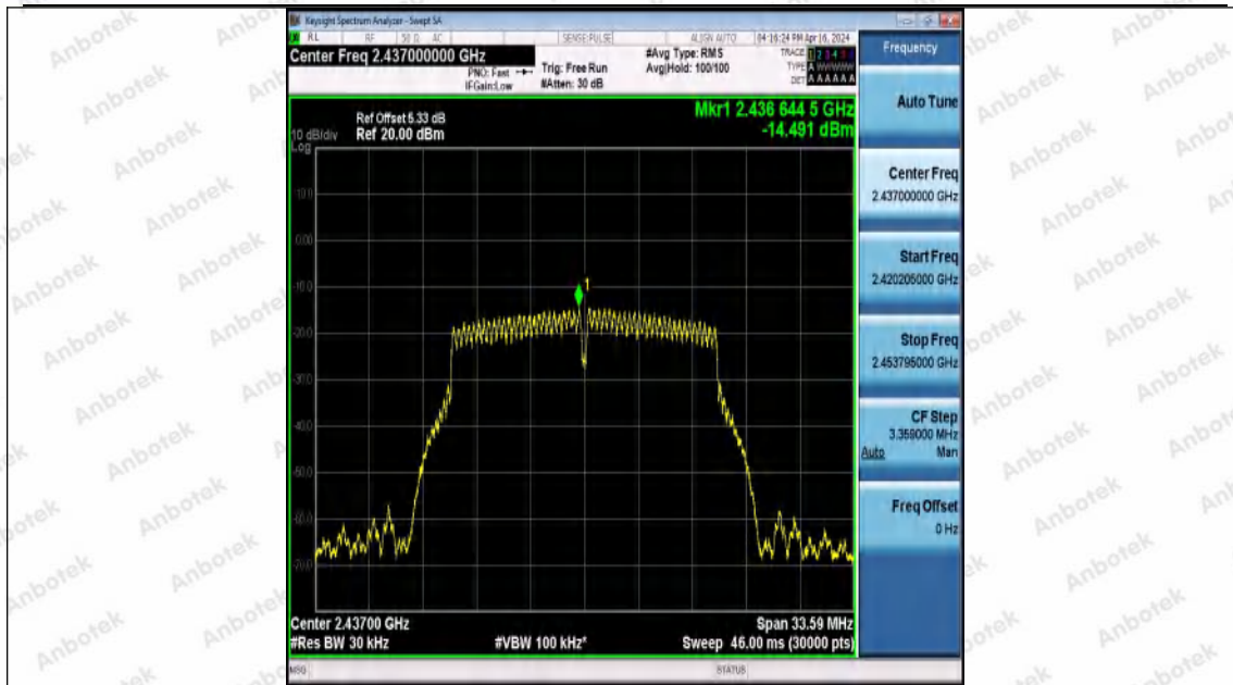
11G-Ant0-2437-PASS
