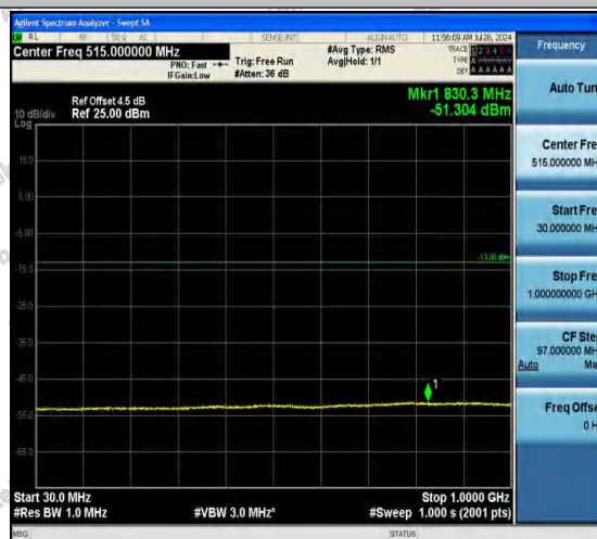
Band2-9538-3-30~1000MHz-PASS
