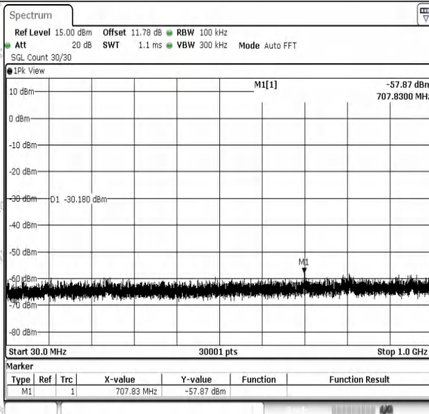
11G-Ant1-2437-30~1000-PASS
