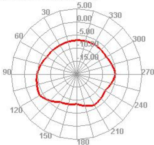
2470.000MHz E2
