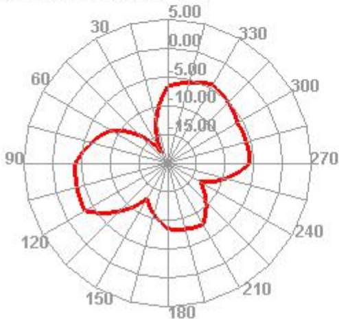
2470.000MHz E1
