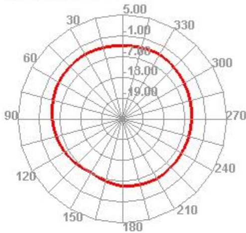
2470.000MHz H
