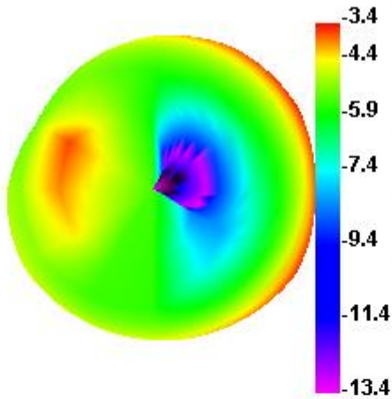
2470.000MHz E1
