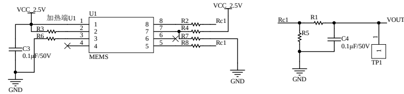
MEMS传感器电路
