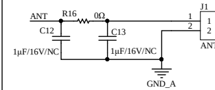
蓝牙天线
