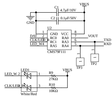
MCU电路
